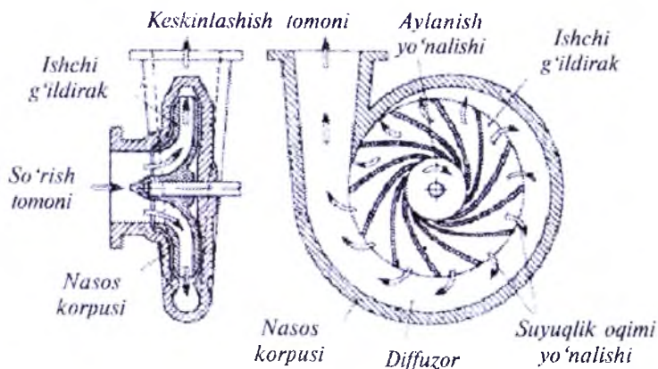
3.7-rasm. Nasos va uning kesimda ko'rinishi.
