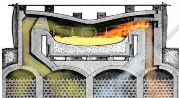
Расми 18. Печи Мартен (бурдашуда).
