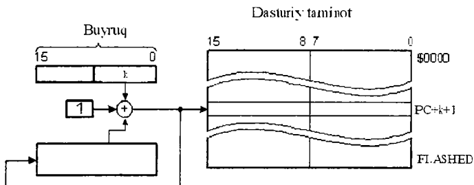
4.29-chizma. Dastur xotirasini nisbatan adreslash
