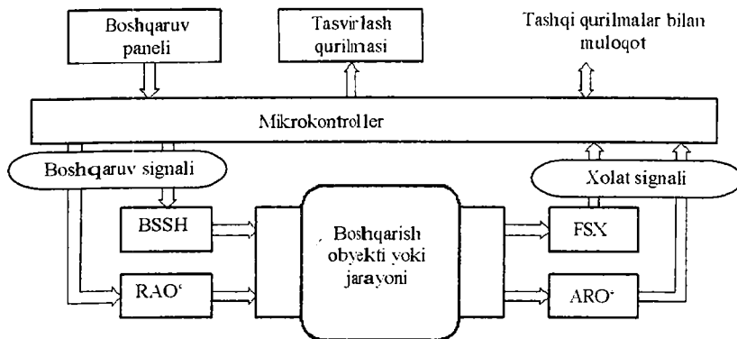
4.1-chizma. Mikrokontroller asosidagi boshqaruv tizimining odatiy tuzilishi: BSSH – boshqaruv signallarini shakllantirgichlar; BQ – bajaruvchi qurilma; D – datchiklar; ShSh – signallar holatini shakllantirgichlar
