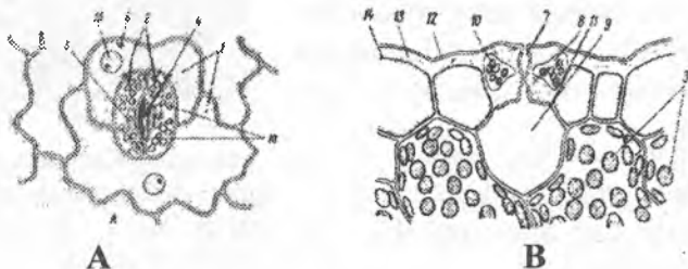
11-rasm. Epidermisdagi ustitsaning tuzilishi: A – ustitsaning ustidan ko‘rinishi, 1 – epidermis hujayrasi, 2 – ustitsaning qamrovchi hujayrasi, 3 – ustitsa teshigi,
