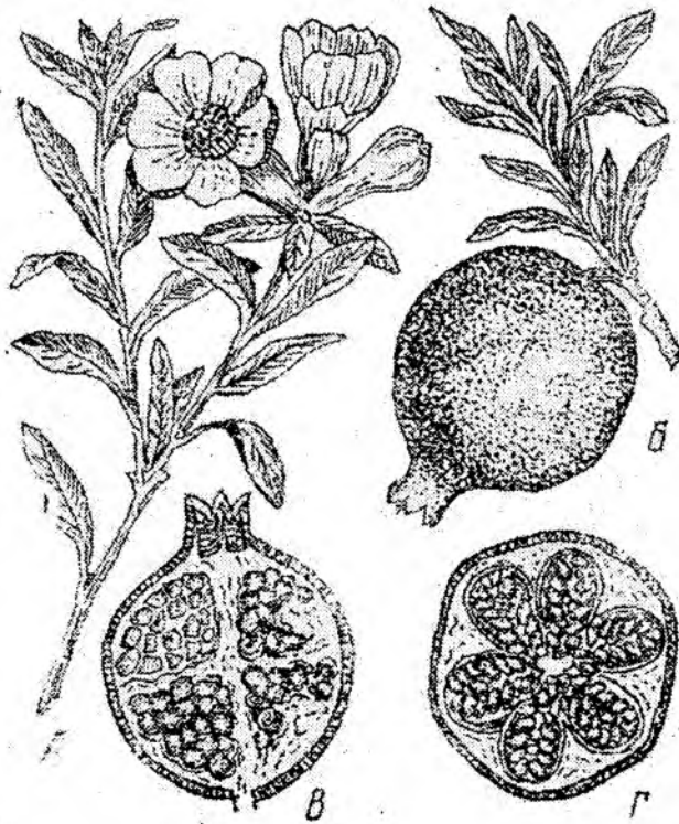
101-rasm. Anor ( Punica granatum ). A – gulli novdasi, B – pishib yetilgan mevasi, V – mevasining biylama kesimi, G – mevasining kandalang kesimi
