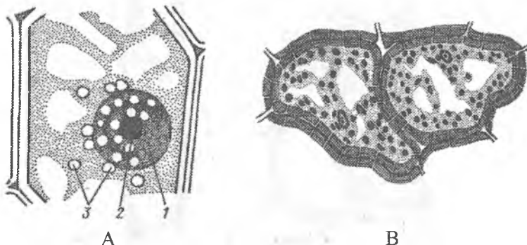
5-rasm. Plastidalar. A - Tradiskansiya barg epidermisi hujayrasi: 1- yadro 2-yadrocha, 3-leykoplastlar. B - Qizil Qalampir mevasi ho'jayrasidagi xromoplastlar
