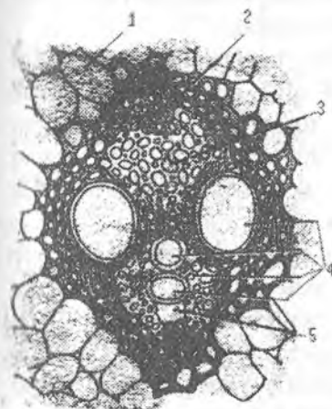
16-rasm. Makkajo'xori poyasidagi yopiq o'tkazuvchi bog'lam.
