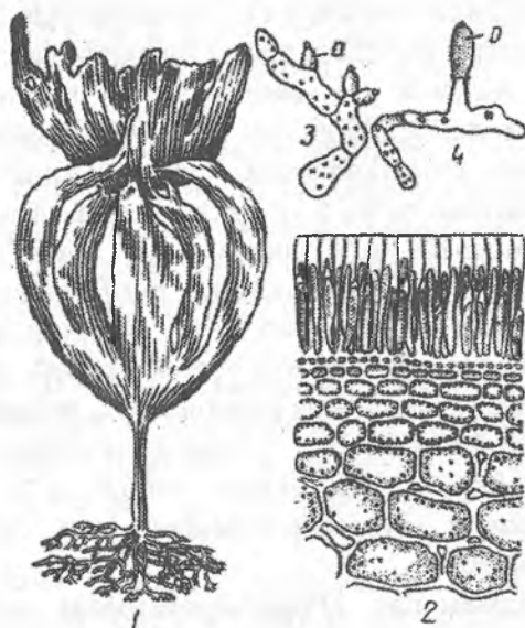
63-rasm. Laminariya ( Laminaria digitata ): 1 – o'simlik bargining almashish payti, 2 – zoosporangiyali bargning kesimi, 3 – anteridiyalı erkak ʻsimtasi (a), 4 – oogamiyalı urg'ochi ʻsimtasi.(b)
