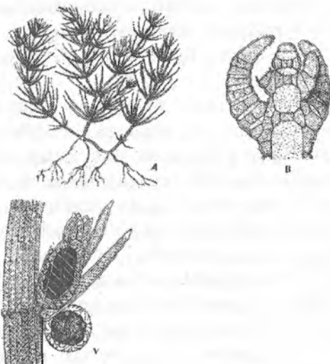
61-rasm. Xara (Chara foetida): A - tallomning umumiy kurinishi, B - ÷sish niqtasining uzunasiga kesimi, V - jinsiy organlarning «poya»da joylashuvi
