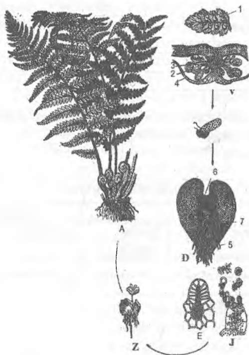
78-rasm. O'rmon qirqqulog'i ( Dryopteris filix mas ):
