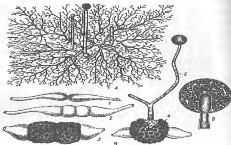
68-rasm. Mukor ( Mucor mucedo ) zamburugʻi: A – zamburugʻ mitsiliyasi va sporangiyaning rivojlanishi, B – yetilgan sporangiya, V – zigotaning hosil boʻlishi, 1 – 3 – jinsiy jarayon va zigotaning rivojlanishi, 4 – zigota, 5- zigotani oʻsishi
