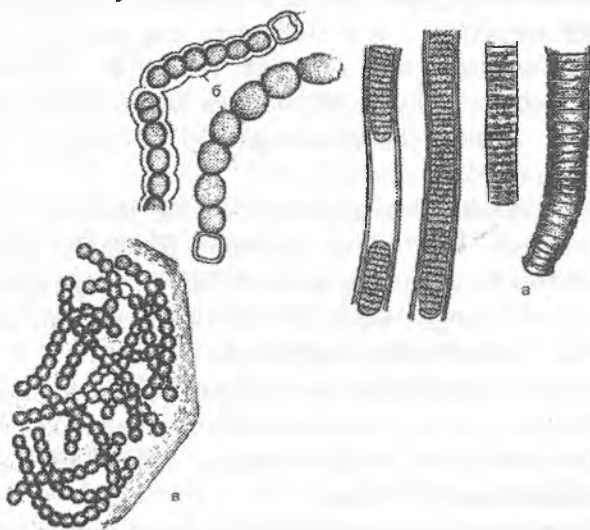
56-rasm. Sianofitaitoifalar. A. a – Nostok (umumiy kùrinishi), b – geterotsistli iplar B. a – ossillatoriya, b – xromotoforali pñst
