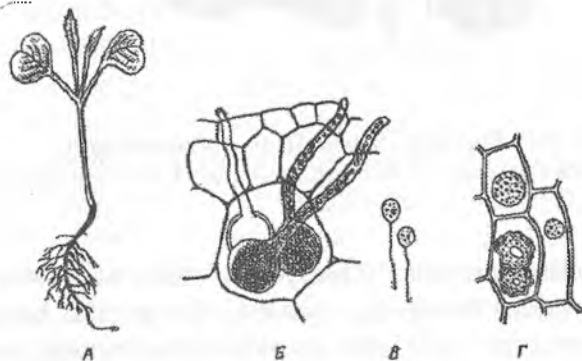
65-rasm. Olpidiy ( Olpidium brassicae ): A - karam kùchatining qoraoyoq (chirish) kasalligi, B – karam tùqimasidagi zoosporangiylar, V – zoosporalar, G – sporangiyanı tınch holatı.
