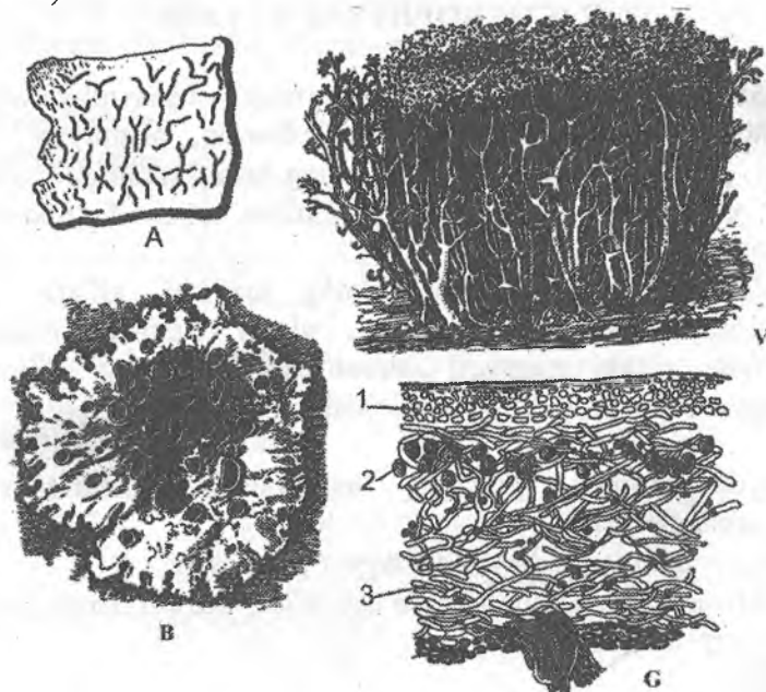
74-rasm. Lishayniklar (Lichenes): A – toshdagi pŕstloqsimon lishaynik, B – bargsimon lishaynik, V – bug‘i lishaynigi, G – lishaynik kesimi: 1 – ustki pŕstloq qavati, 2 – gonidiyali qavat, 3 – zambrug‘ gifasi, 4 – ostki po‘stloq qavati.
