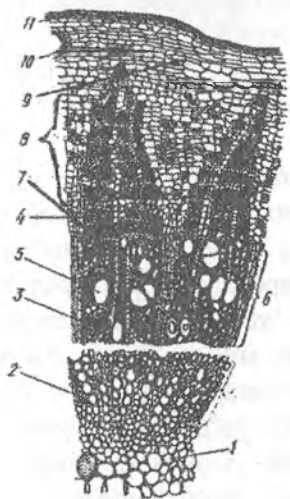
33-rasm. G'oz poyasining ichki tuzilishi: 1 - o'zak, 2 - birlamchi ksilema, 3 - yog'ochlik tolalari, 4 - o'zak nuri, 5 - suv naylari, 6 - ikkilamchi ksilema, 7 - kambiy, 8 - ikkilamchi floema, 9 - po'stloq parenximasi, 10 - ajratuvchi sistema, 11 - periderma.
