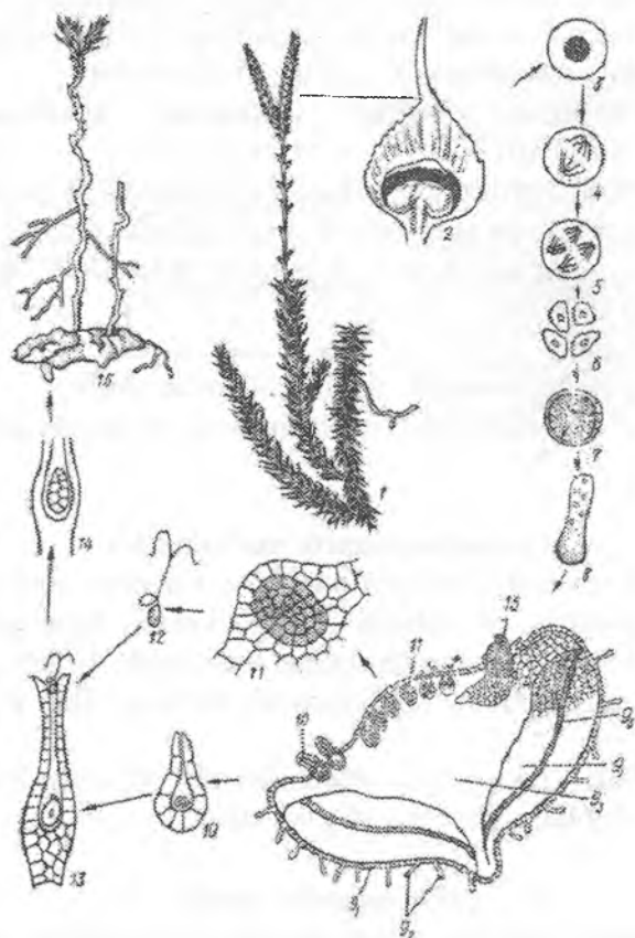
76-rasm. Cho'qmoqli plaun ( Lycopodium Slavatum ) ning rivojlanishi: 1 - Sporafit, 2 - sporafil sporangiyasi bilan, 3 - 6 - sporangiya xujayrasidagi sporaning meyoz yili bilan rivojlanishi, 7 - spora, 8 - sporaning usib protonimani xosil qilishi, 9 1 - 9 5 - arxegoniyali va anteridiyali gametofit, 9 1 - epiderma, 9 2 - rizoid, 9 3 - parinxima, 9 4 - ustunsimon qavat, 10 - arxegoniya.
