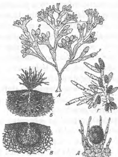
64-rasm. Fucus ( Fucus ): A – umumiy kurinishi; 1- havo pufakchasi, 2 – konsen-takullar, B – ooganiyli skafidiy, V – sper-matozoidli skafidiy, G – anteridiyli tallomning bir qismi, D – oogoniy
