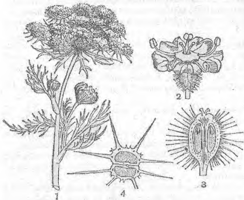
84-rasm. Sabzi ( Daucus carota ). 1 – tūpguli, 2 – guli, 3 – mevasining uzunasiga kesimi, 4 – mevasinng kūndalang kesimi
