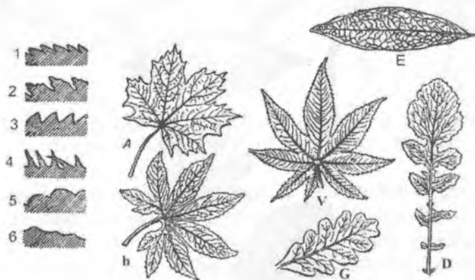
37-rasm. Oddiy barg xillari: A – bo'lma barg, B – qirqilgan barg, V – bo'lingan barg, D – lira-simon barg, E – lansetsimon barg. 1 – arrasimon qirrali, 2 – ikki marta arrasimon qirrali, 3 – tishsimon qirrali, 4 – o'tkir tishsimon qirrali, 5 – kungurasimon qirrali, 6 – chuqursimon qirrali
