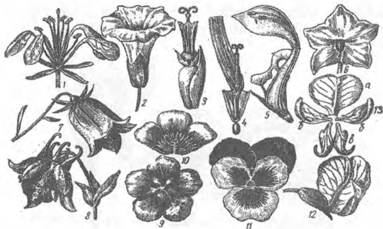
46-rasm. Har xil shaklli gultojlar: 1, 2, 3, 6, 7, 8, 9, 10 – to'g'ri – aktinomorf gullar, 4, 5, 11, 12 – noto'g'ri – zigamorf gullar, 13 – gulning alohida qismlari: – a – elkan, b – kurakcha, v – qayiqcha.
