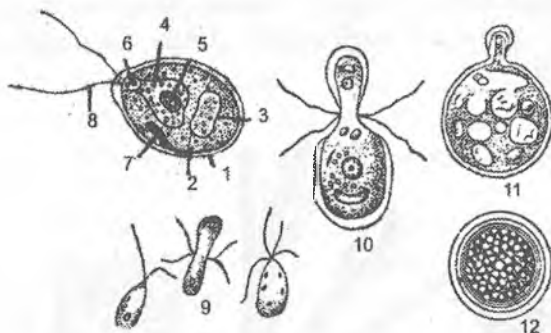
57-rasm. Xlamidomonada (Chlamydomonas)ning tuzilishi va jinsiy k payishi: 1 – pektin moddali po'st, 2 – sitoplazmasi, 3 – perinoid, 4 – xromoto-forasi, 5 – yadrosi, 6 – vokuolasi, 7 – ko'zchasi, 8 – hivchin, 9 – izogametalarining qushilishi,
