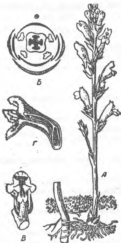
89-rasm. Shumgiya ( Orobanche ramosa ): A – o‘simlikning ildizida parazitlik qilayotgan shum‘riya, B – gul diagrammasi, V – guli, G – gulning b‘yig‘a kesimi
