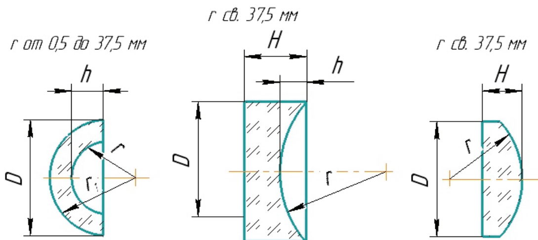
Рис. 171. Виды рабочих пробных стекол
