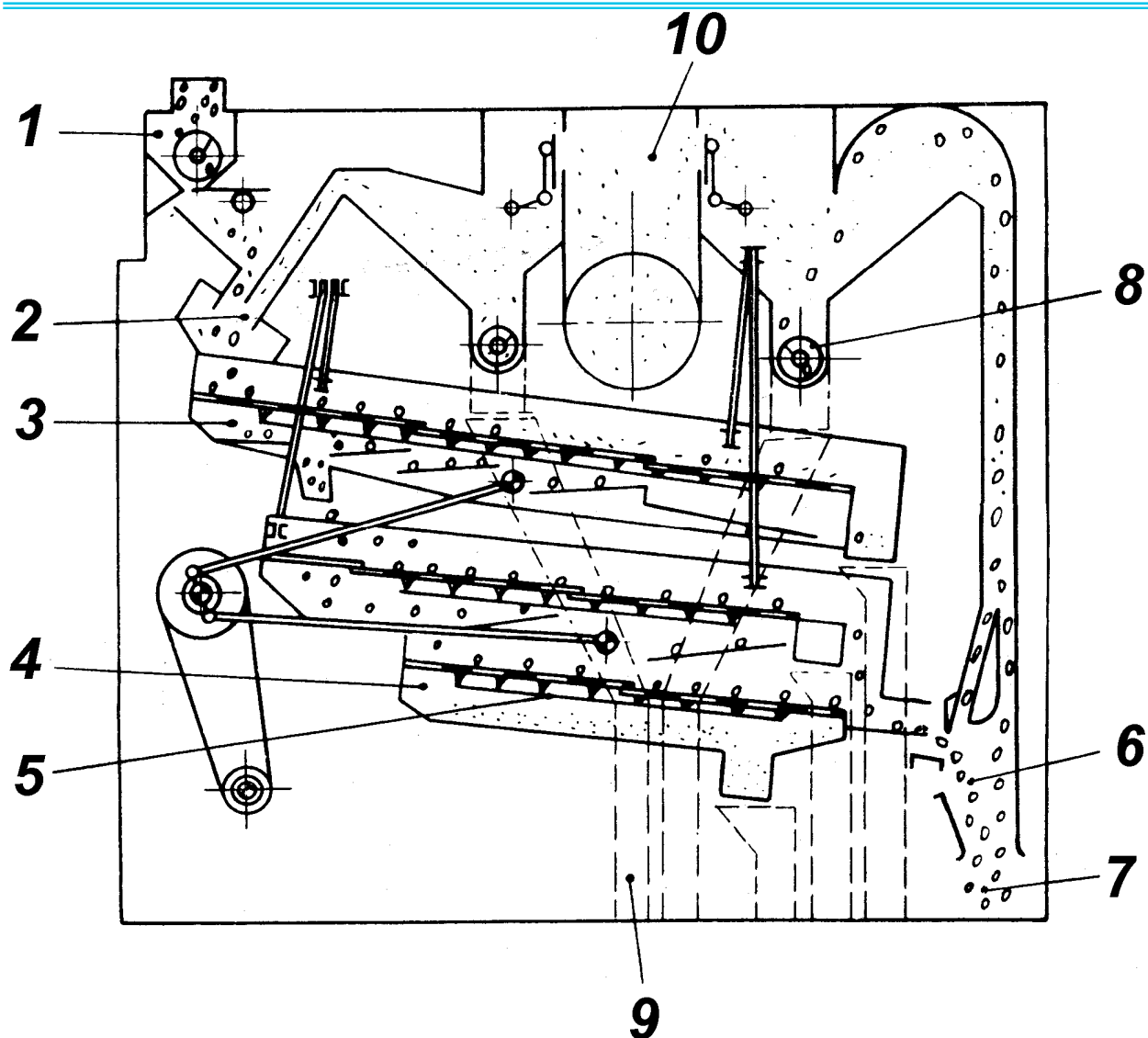
10- rasm. K-547 (Petkus) chigit tozalash mashinasining sxemasi
