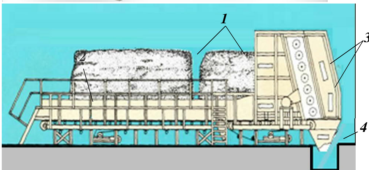
17-Rasm. Qo‘zg‘almas paxta moduli buzgich
