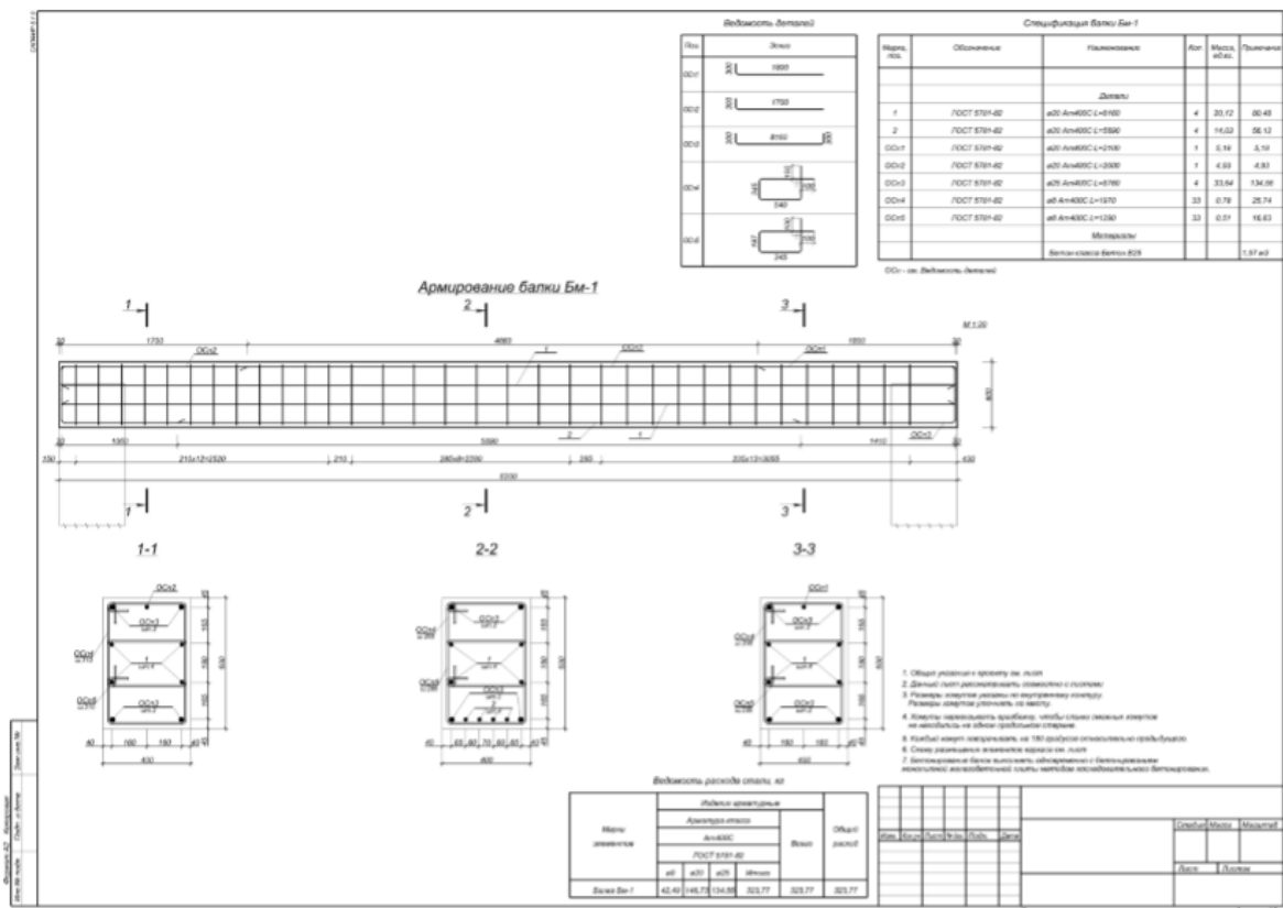
42–rasm. To‘sinni armaturalash chizmasi.
