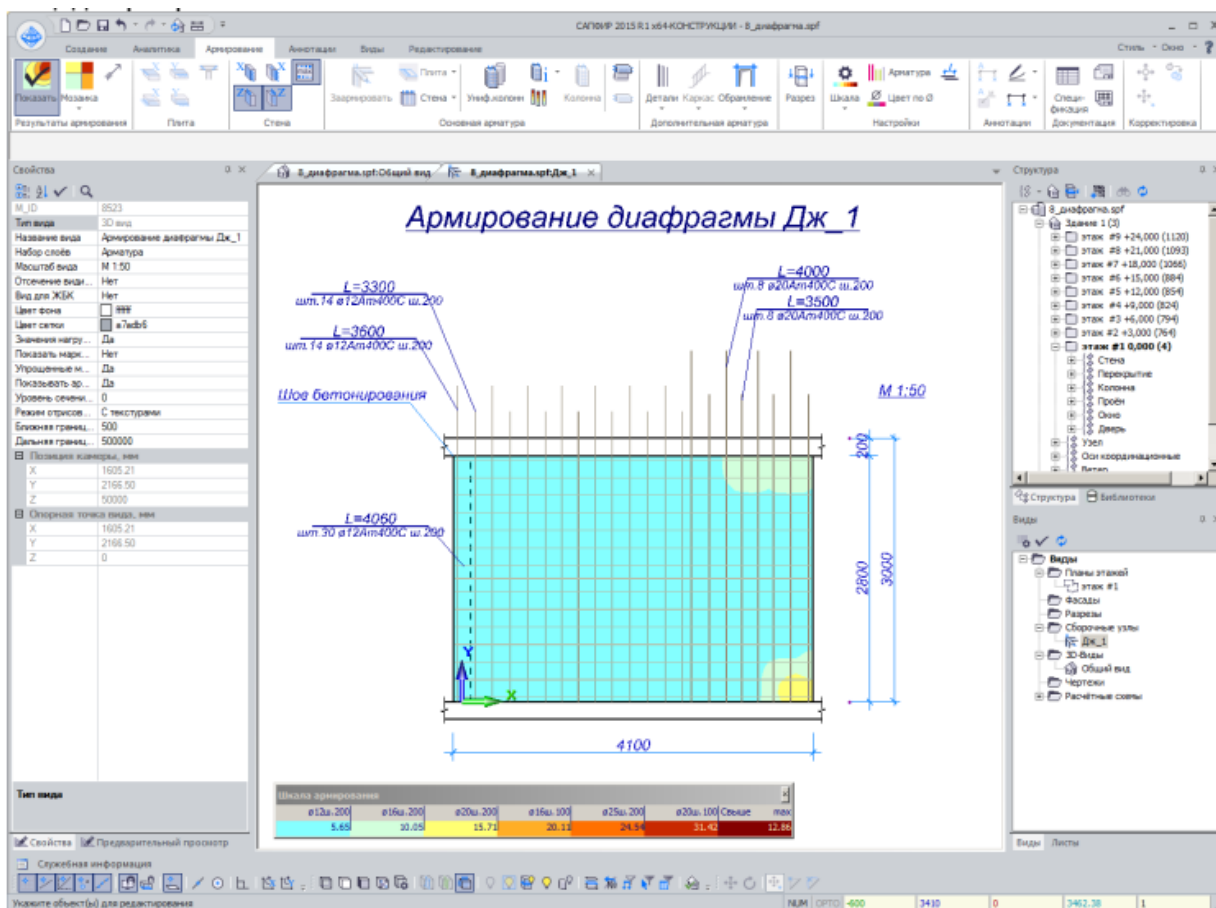
52-rasm. DJ_1 diafragmani avtomatik konstruksiyalash
