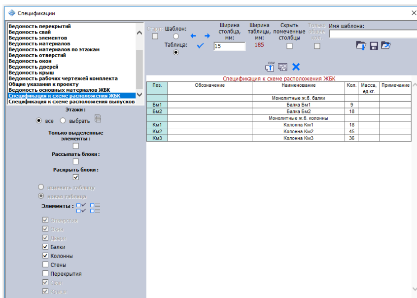
27-рasm. Spetsifikatsii muloqat oynasi
