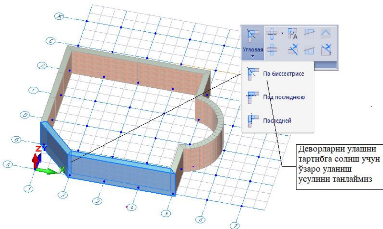
5-rasm. Devor fragmentlarini qirqish va ulash
