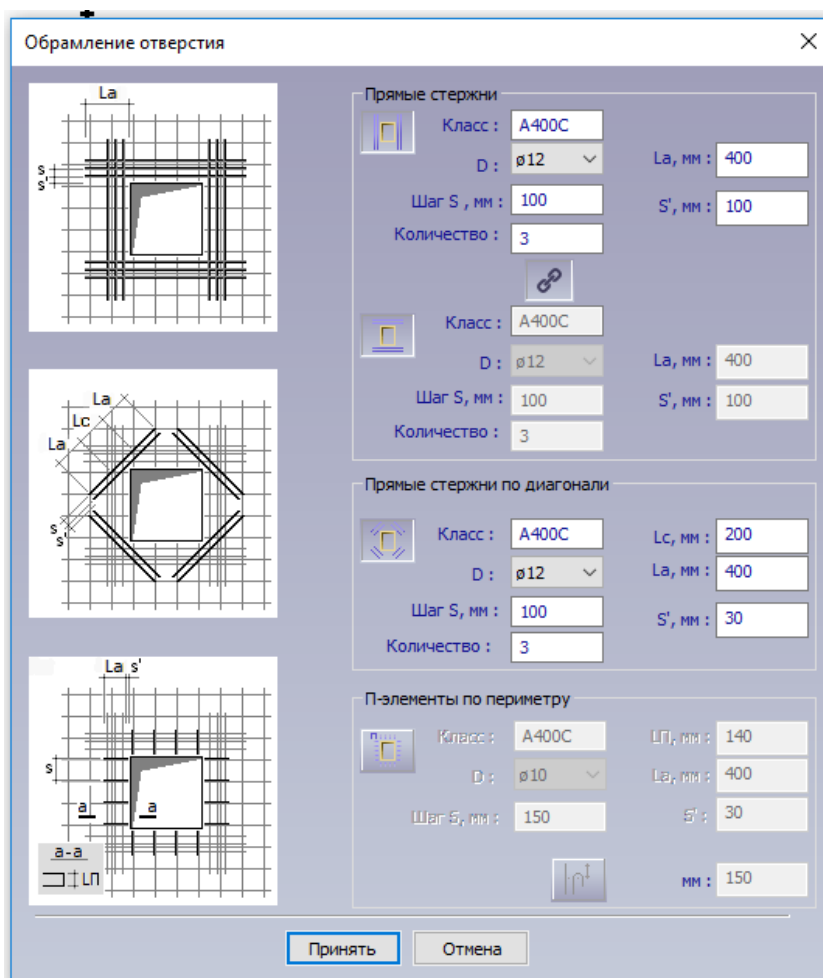
62-rasm. Обрамление отверстия muloqat oynasi
