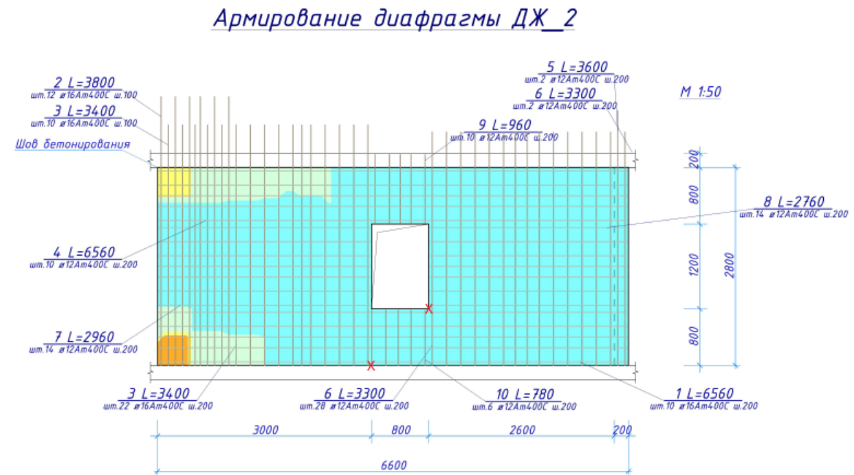
58-rasm. Deraza ostida armaturalash zonasini joylashtirish
