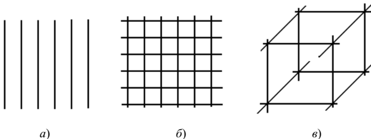
Рис.1. Схемы армирования: а – одноосное; б – двухосное; в – трехосное (объёмное)
