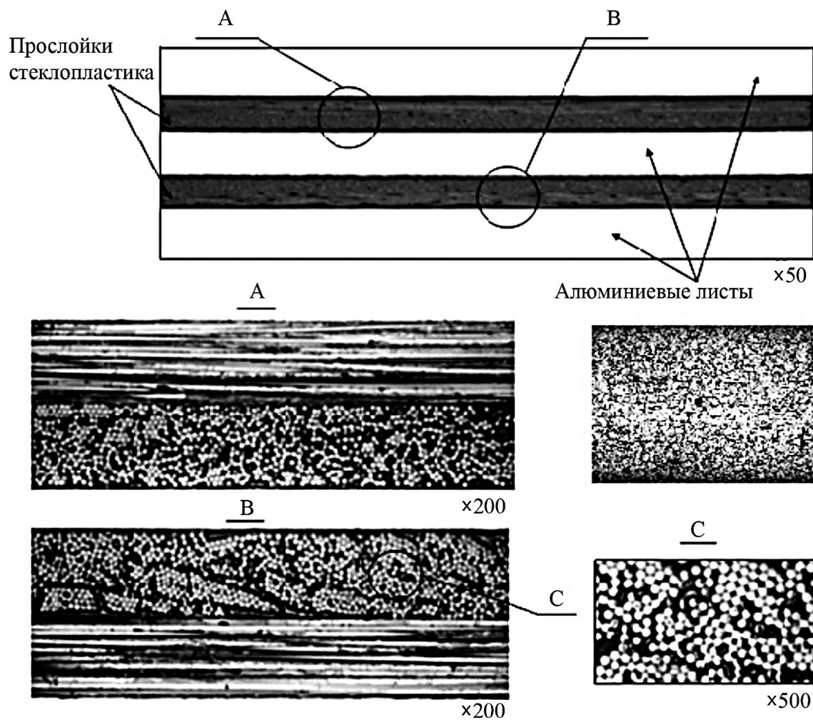
Рис. 1. Типичная микроструктура 1441-СИАЛ-3-1 пятислойного строения (3/2) с перекрестным армированием (0/90) слоя пластика
