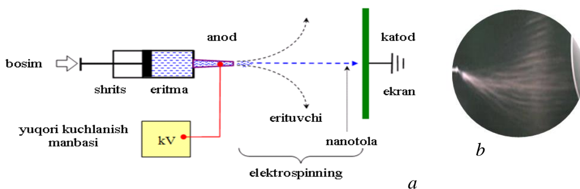
2-rasm. Elektrospinning prinsipial chizmasi (a) va elektr maydonida fileradan chiqayotgan polimer suyuq fazali oqimdan erituvchini sochilishi va makromolekulalarni orientatsion eshilgan holga nanotolalar bo‘lib shakllanib ekranga borib tushishining fotosurati (b)
