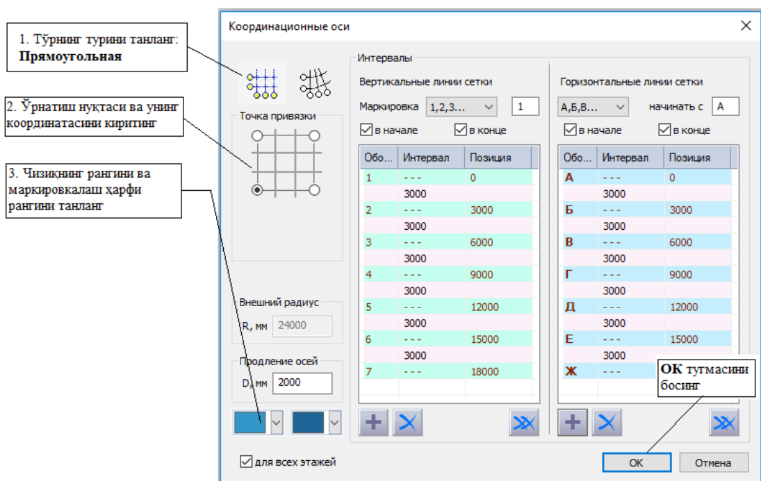
1-rasm. Koordinatsiya o‘qlari muloqat oynasi
