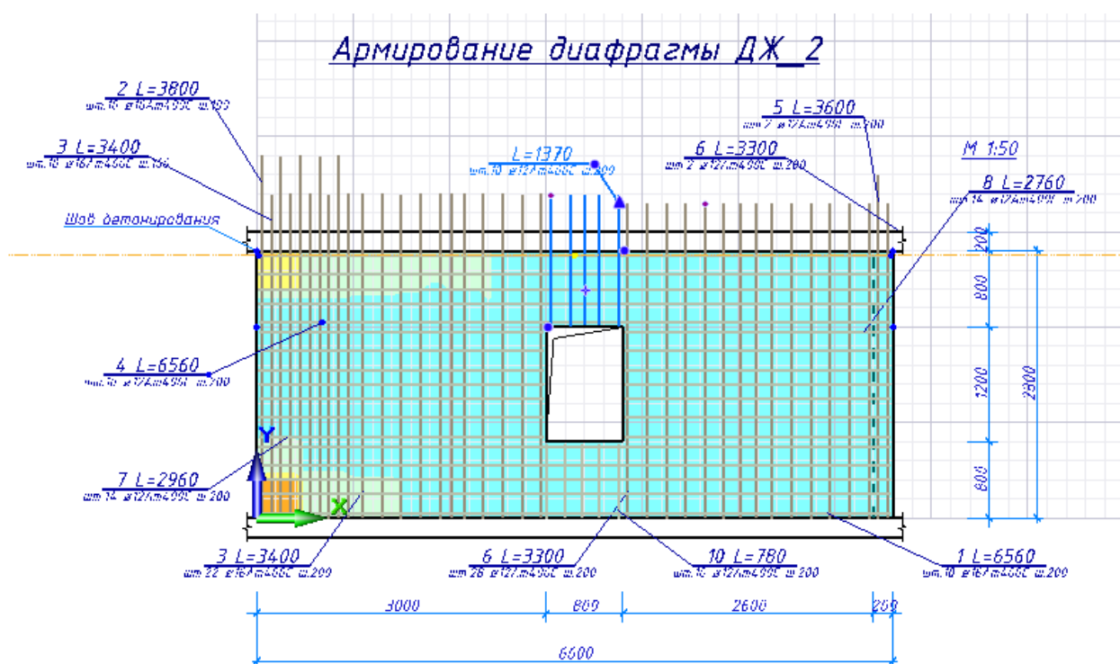
13.17-rasm. Armaturalash zonasi uchun chiqiq uzunligini tahrir qilish
