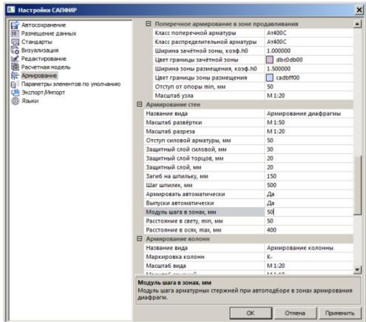
13.16-рasm. Настройки САПФИР мулоқот oynasi
