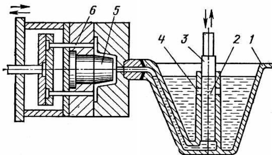
3.7-rasm. Issiq kamerali presslaydigan mashinalarda quyma tayyorlash jarayonining sxemasi
