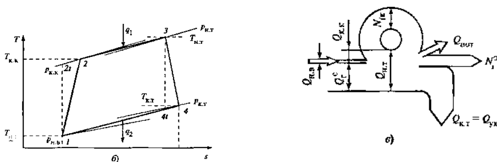
Рис. 1.3. Принципиальная схема одноступенчатой газовой турбины.
