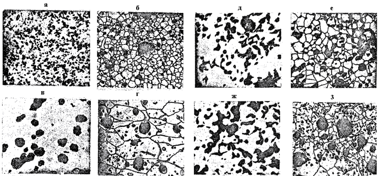
4.5-rasm. Oksid magniy asosli keramik materialning mikrostrukturasi
