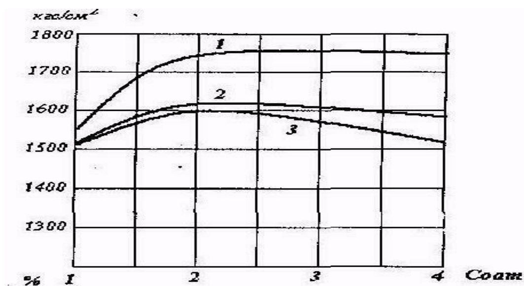
2.6-rasm. Qizdirib pishirish temperatura va vaqtining materialning mexanik xossasiga ta'siri: 1-1500°C, 2-1800°C, 3-2000°C.
