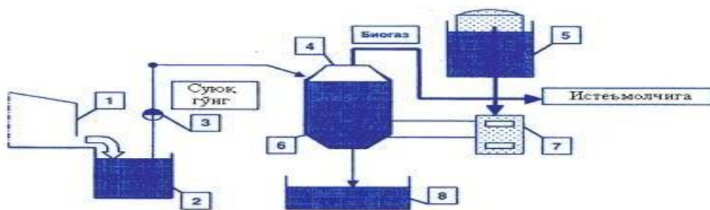
1-чизма. Биогаз ишлаб чиқариш технологияси Гўнг шарбатини биогаз ускурмасида қайта ишлашни технологик чизмаси
