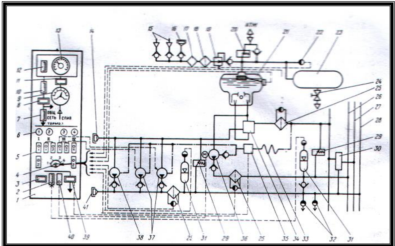
Рис 6. Схема сети источников давления и панель гидросистемы.
