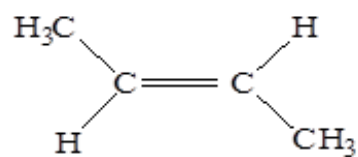
транс-бутен-2
