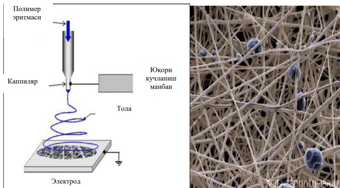
5.36-расм. Электроспиннинг методи асосида тола тайёрлаш қурилмасини схемаси
