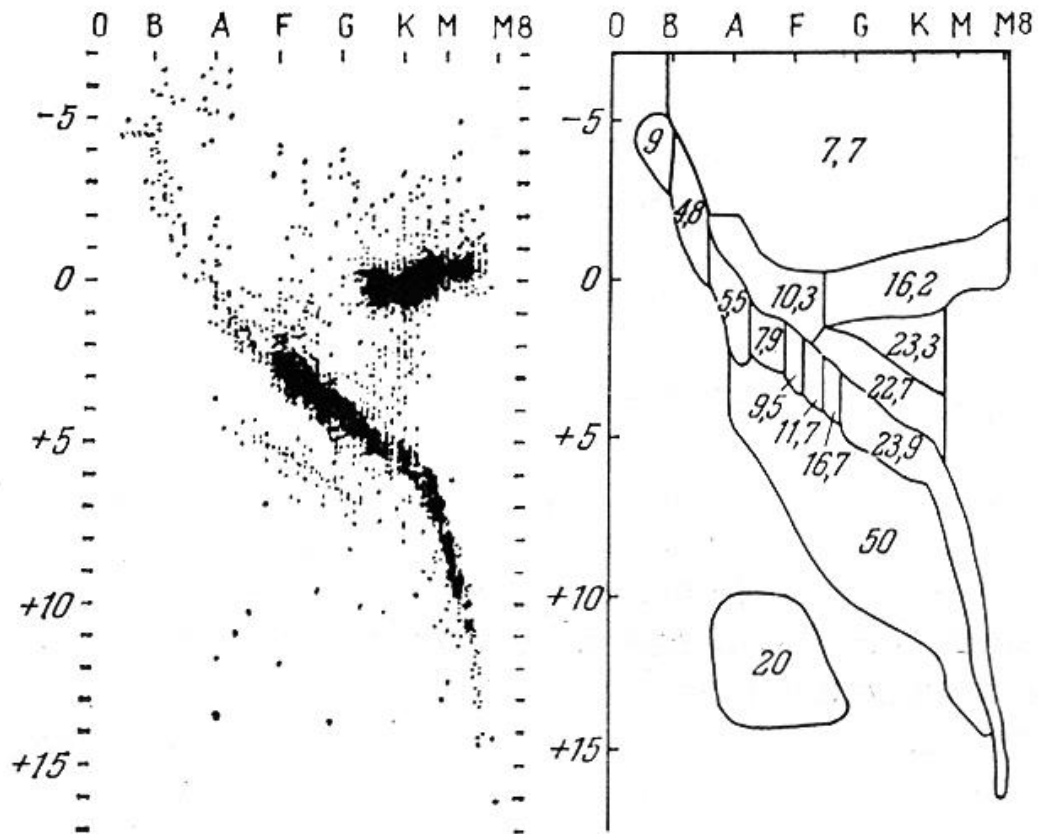
расм-7. Гершпрунг-Рассел диаграммаси ва айрим юлдузлар гуруҳларининг фазовий харакат тезликлари
