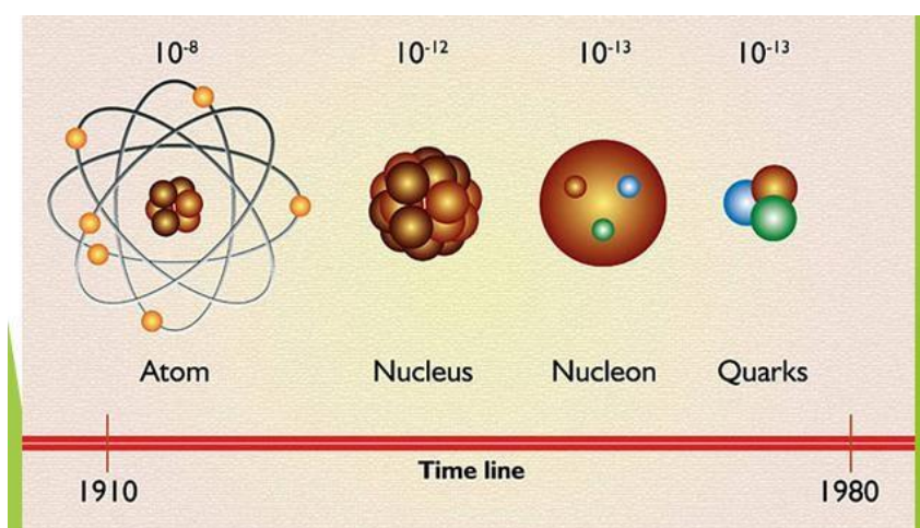
3-расм. Табиатдаги элементар зарралар.
