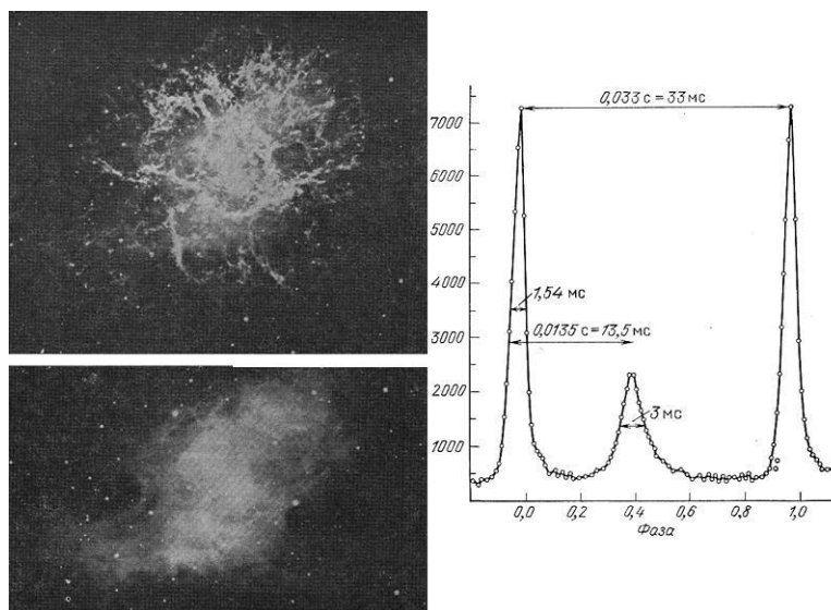
10-расм. Қисқичбақасимон туманлик ва унинг ичида кузатиладиган пульсарнинг интенсивлигини ўзгариш чизиги.
