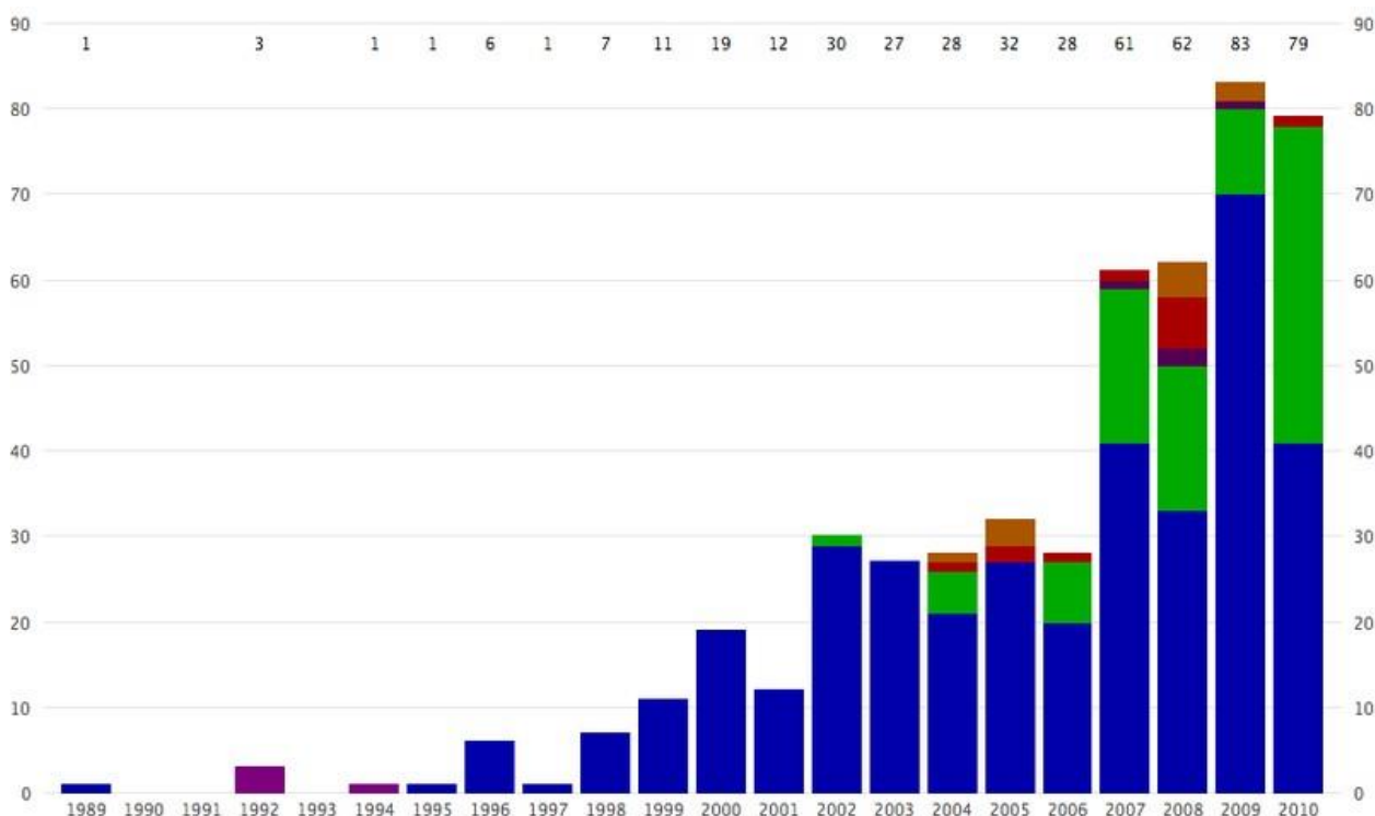
Шакл.1. 1989-2010 йилларда экзопланеталар кашфиётининг хронологияси Мовий - спектроскопик кашфиётлар, яшил - фотометрик кашфиётлар (транзит усули). Қолган ранглар (декодлашсиз, кашфиётларнинг умумий сонининг тахминан 5%) тўғридан-тўғри суратга олиш (12 кашфиёт), микроленсия (10 кашфиёт), радио пулсарларидаги вақт ўзгариши (4 кашфиёт) ва вақтинчалик ўзгариш каби кашфиёт усулларини бирлаштиради. бошқа юлдузлар (4 кашфиёт).
