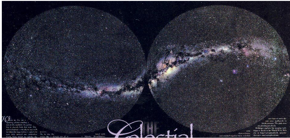
1-расм. Осмон сферасининг шимолий (чапда) ва жанубий (ўнгда) яримшарларида Сомон йўлини кўришиши.
