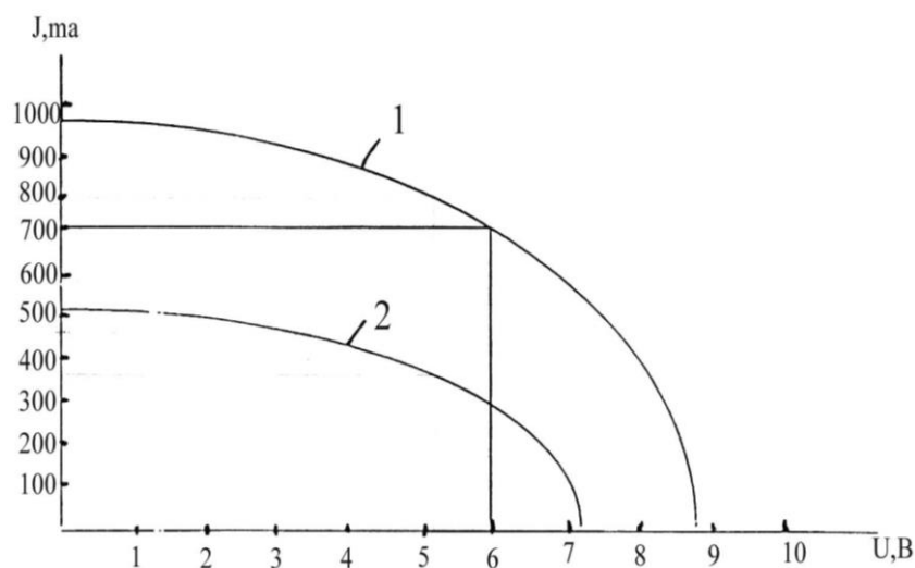
1.2-расм. Ясси қуёш батареясининг вольт-ампер тавсифи.
