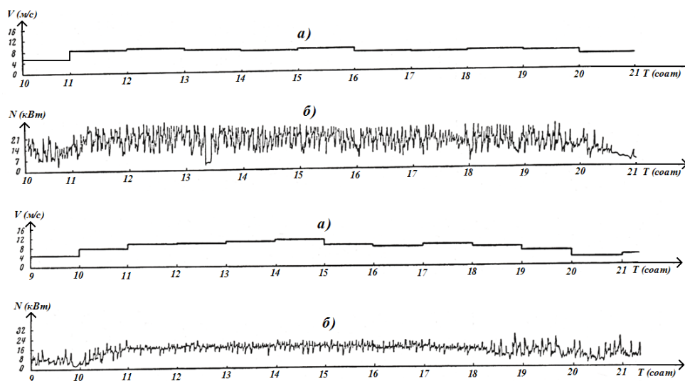
4.6-расм. Шамол электростанциясининг ишлаш графиги:
