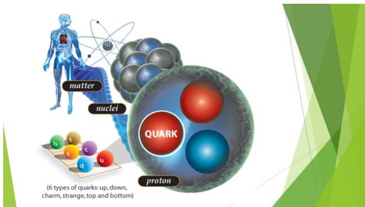
1- Расм. Инсоният қуйи йўналишида ҳаракатланиб (молекула – атом – ядро – протонлар, нейтронлар - кварклар) инсон кичик масофалардаги жараёнларни тушунишга ҳаракат қилди
