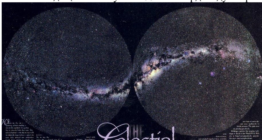
1-расм. Осмон сферасининг шимолий (чапда) ва жанубий (ўнгда) яримшарларида Сомон йўлини кўриниши.
