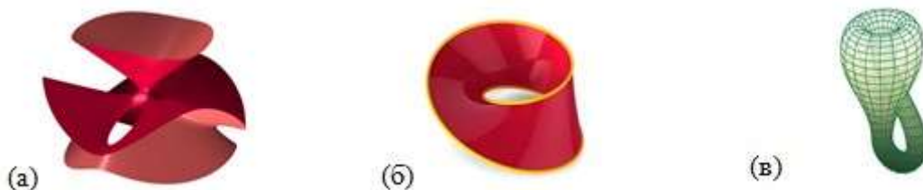
2-расм. Буюртманинг алгебраик юзалари 2 дан катта: (а) Диагонал куб Слебсч юзаси, (б) Мобиус тасмаси, (с) Клеин шишаси.
