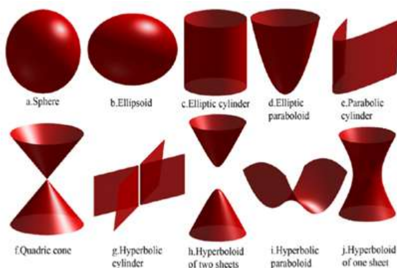
1-расм. 2-тартибли алгебраик юзалар
