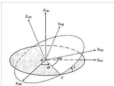
Эйлер бурчаклар
