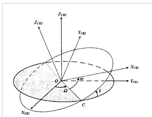
11-расм. Эйлер бурчаклари
