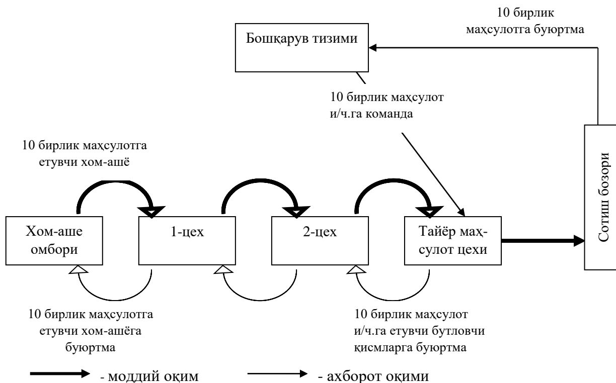
13-расм. Ишлаб чиқариш логистикасида моддий оқимларни бошқаришнинг «тортувчи» тизими
