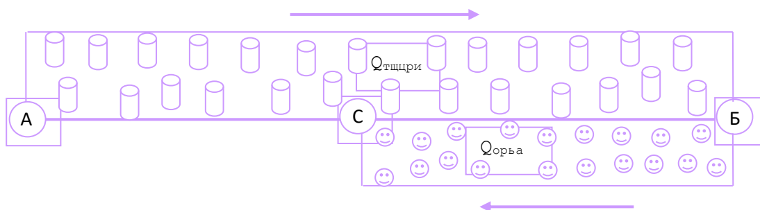
35-расм. Орқа томонга қисман юкли маятник маршрут чизмаси
