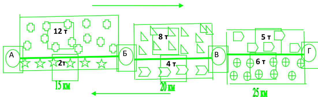
33-расм. Тарқатиш маршрути чизмаси
