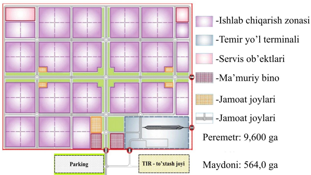
26-расм. “Навоий” эркин индустриал иқтисодий худудининг схемаси: Навоий шаҳар аэропортининг юк терминалигача бўлган масофа-1,8 км; т/й разъездигача бўлган масофа-3 км; “Е- 40” автомагистралигача бўлган масофа- 0,8 км.
