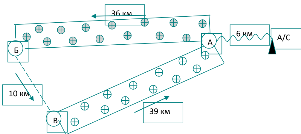
29-расм. Бир томонга оғувчи маятник маршрут чизмаси
