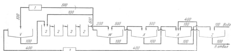
Рис. 68. К расчету схемы непрерывной противоточной декантации:
