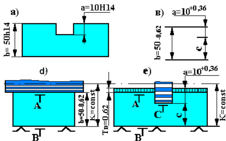
5-rasm. Konstruktorlik bazaga mos tushmagan tayanch texnologik B bazadan ariqcha frezalash
