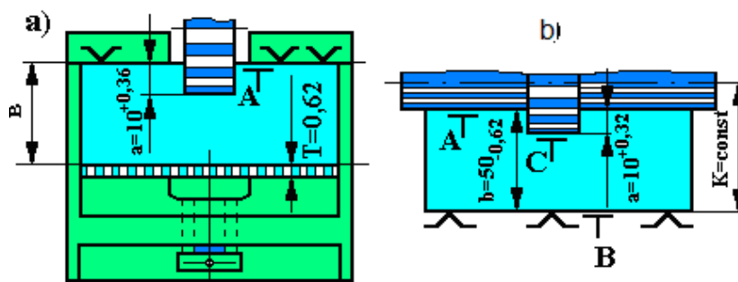
5-rasm. Konstruktorlik bazaga mos tushmagan tayanch texnologik B bazadan ariqcha frezalash
