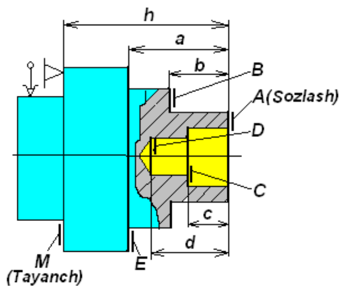
8-rasm. Texnologik jarayonlarni loyihalashda texnologik bazalarni tayinlash sxemasi
