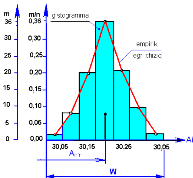
1-rasm. O'lchangan detallar o'lchamlarining o'lchamlarini taqsimlanishi ham turli taqsimoti
