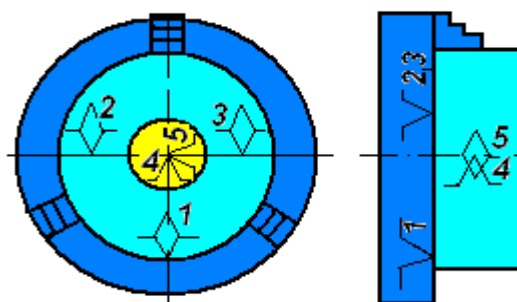
1-rasm. Bazalash prinsiplari: detalda yuzalarida oltita tayanch nuqtalarni joylashtirish sxemalar, 1,2,3 - o'rnatish bazalari, 4,5 –yo'naltiruvchi bazalar, 6 – tayanch bazalari
