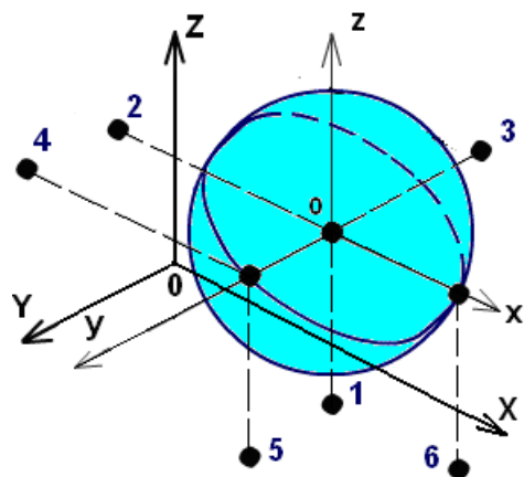
1-rasm. Bazalash prinsiplari: detalda yuzalarida oltita tayanch nuqtalarni joylashtirish sxemalar, 1,2,3 - o'rnatish bazalari, 4,5 –yo'naltiruvchi bazalar, 6 – tayanch bazalari
