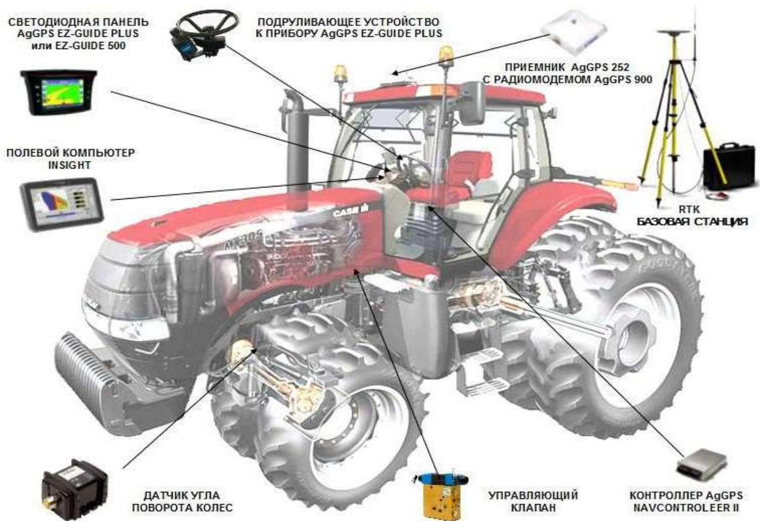
Рис. 12. Параллел харакатланиш ва автопилотлаш курилмаларининг тракторда жойлашиши
