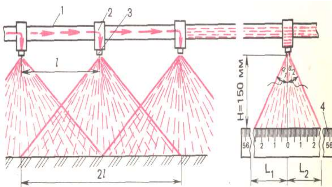
51-расм. Штангали тарқатиш қурилма.
