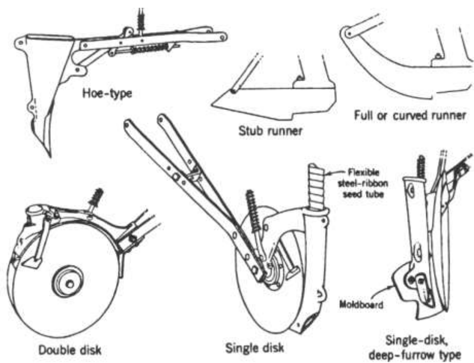
39-расм. Хориж сеялаларининг экичлари.
