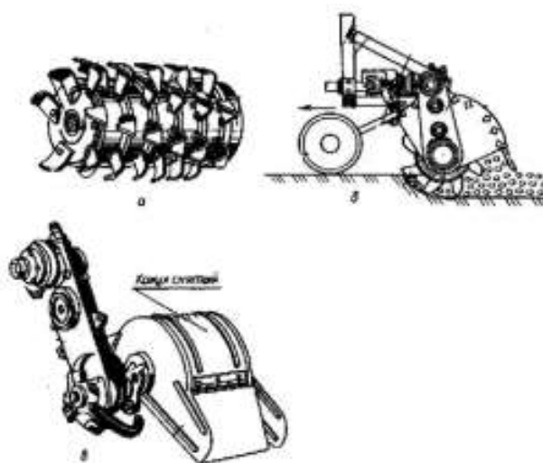
16-рasm. Тупроқ фрезаси.
