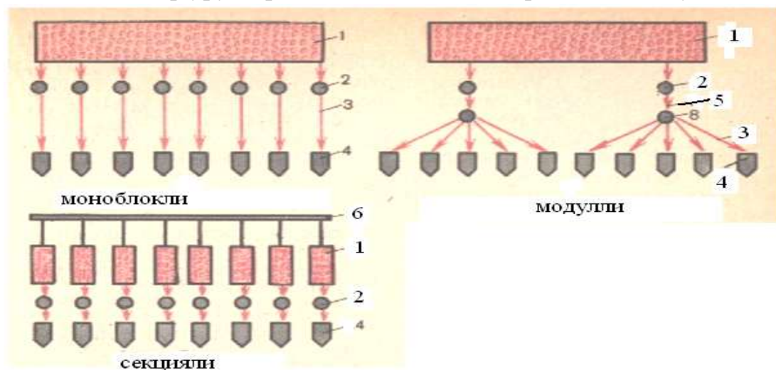
24-расм. Сеялка ишчи қисмларини жойлаштириш схемаси.
