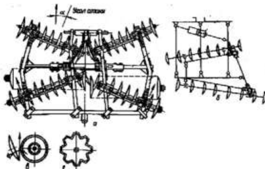
15-рasm. БДН–3 дискли тирма.
