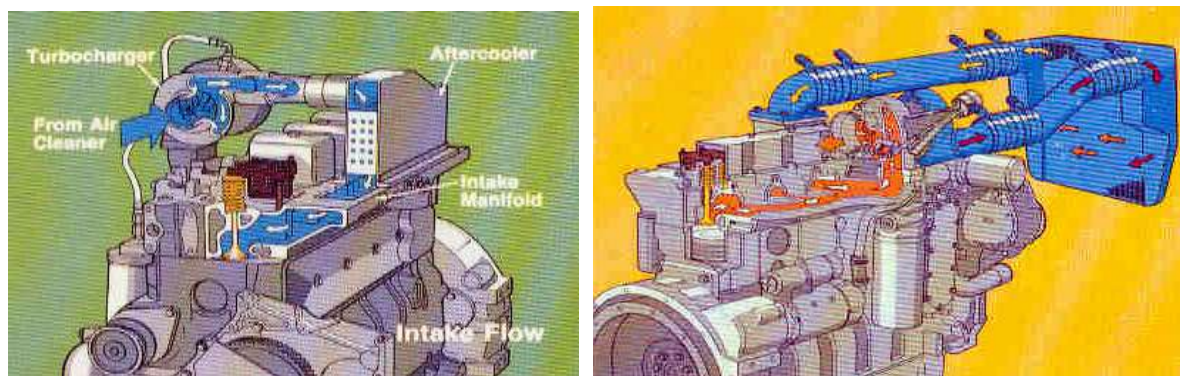
5-расм. Цилиндрларга босим остида киритилаётган ҳавони оралик совитгичлар 17,18
