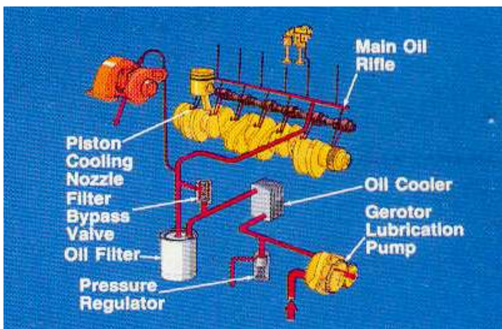
2-расм. Двигател мойлаш тизими элементлари 12
