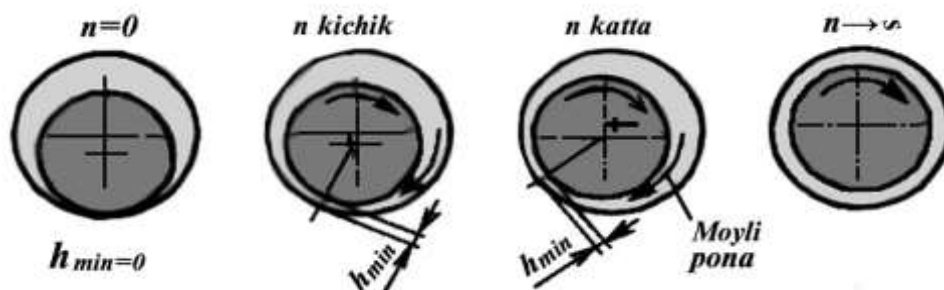
1-расм. Вал ва подшипник бирикмасида мой понасининг ҳосил бўлиши
