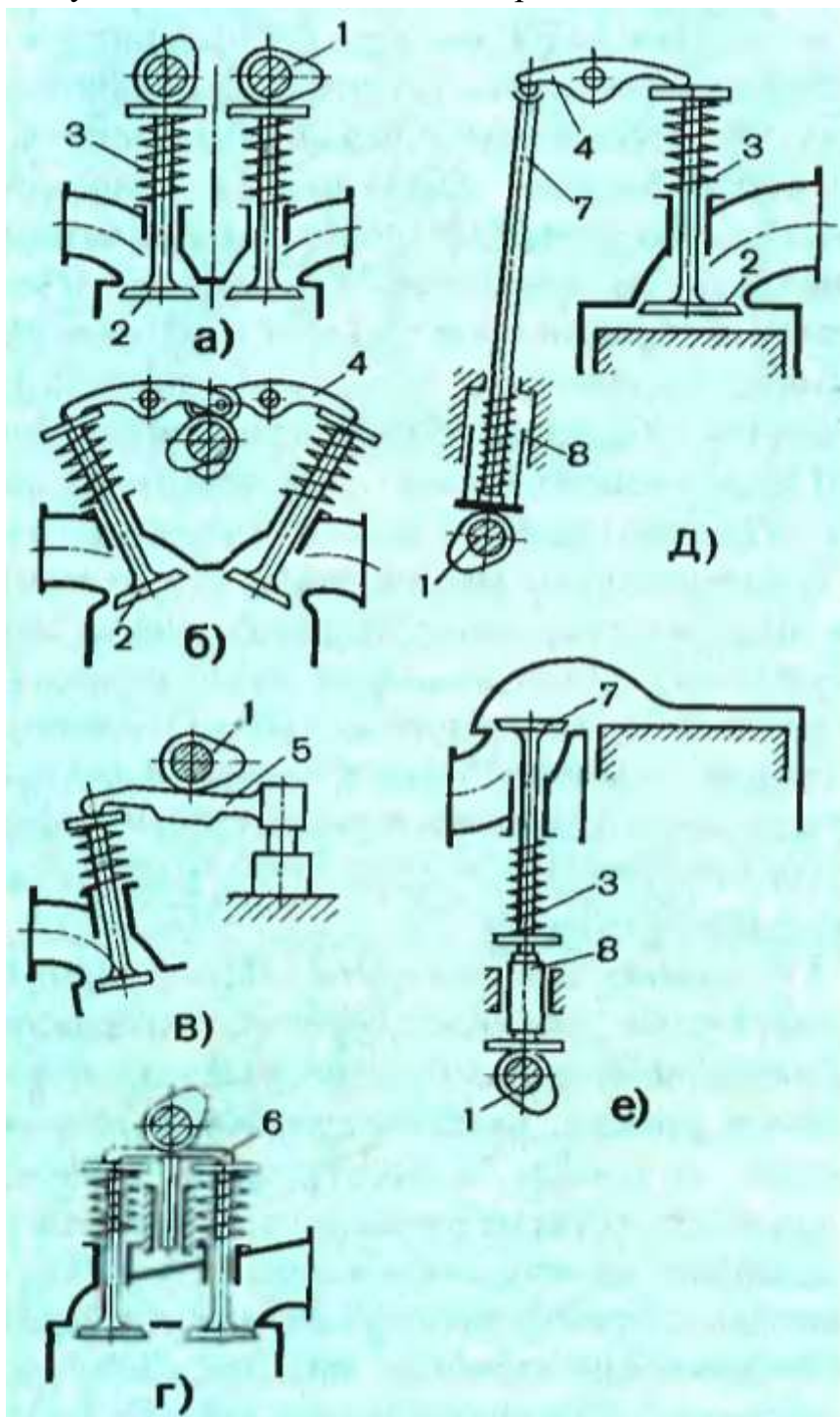
5-расм. Клапанларни ўрнатиши ва уларни ҳаракатга келтириши учун қўлланилган газ тақсимлаш механизми схемалари:
