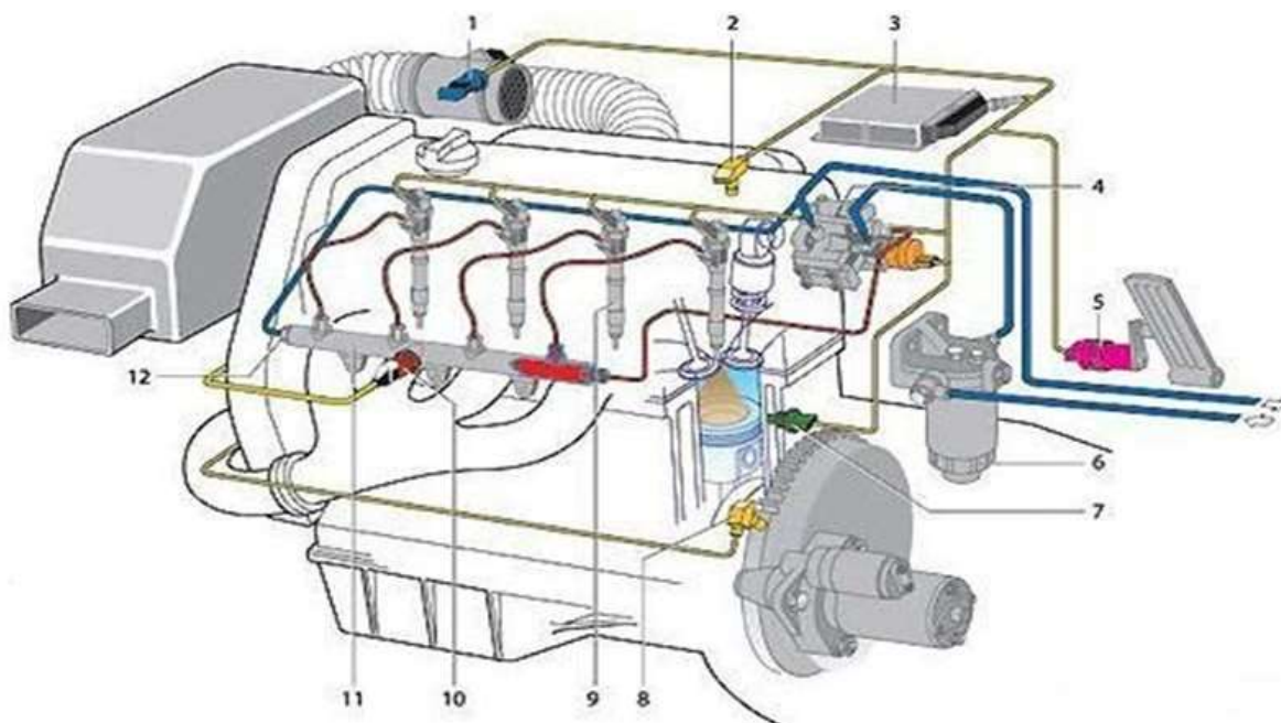
10-расм. Common Rail ёнилғи узатиш тизими элементлари
