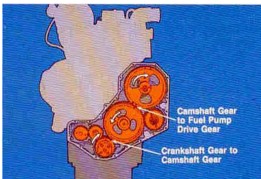
4-расм. Двигателда валларни ҳаракатлантирувчи шестерняларни жойлашиши 8
