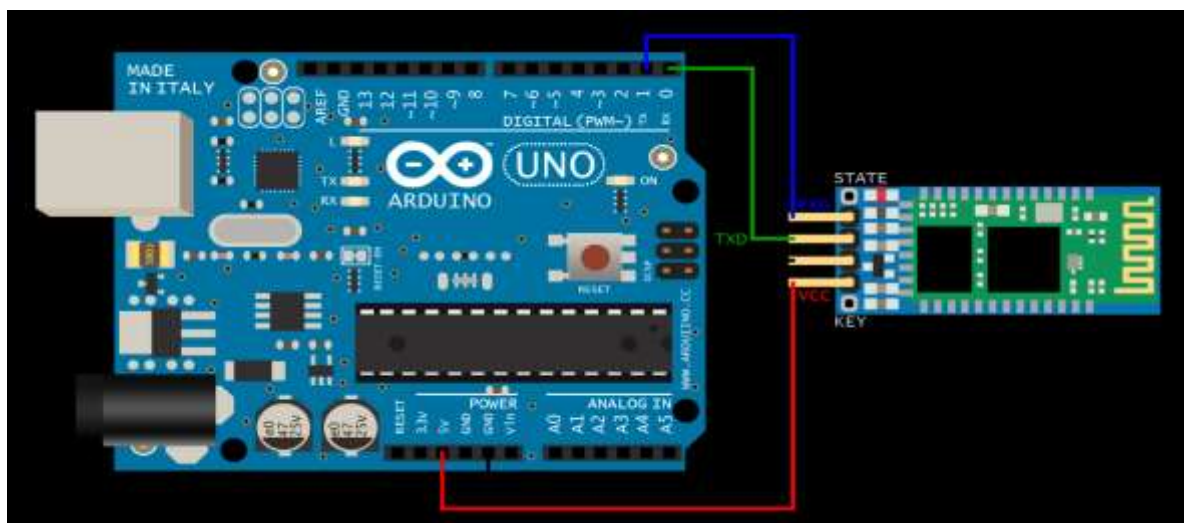
Bluetooth модулини ARDUINO платасига улаш
