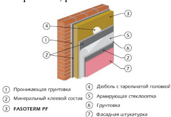
Рис. 4.2. Утепление фасада теплоизоляционной системой с тонкослойной штукатуркой
