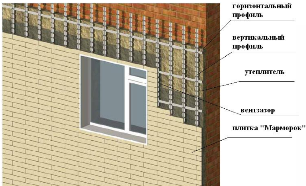
Рис. 4.8. Конструктивное решение системы «Мarmorок»
