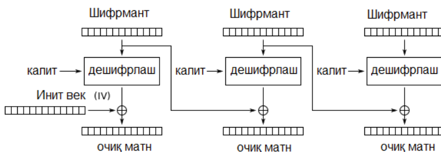
1.14-расм. CBC моделда дешифрлаш
