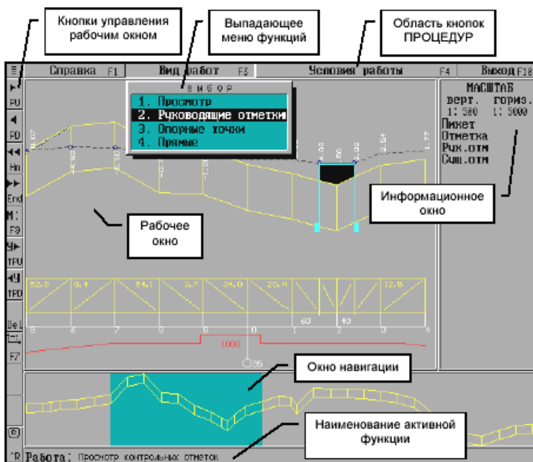
12-расм. Берилган маълумотларни график таҳрир қилишнинг ишчи мухити
