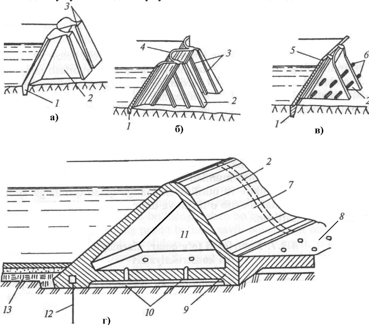
4.2. – расм. Контрфорсли тўғон турлари: а), б), в) - пойдевор плитасиз: а) - массив контфорсли; б) - кўпарқали; в) - ясси ёпмали; г) - пойдевор плитали (ясси ёпмали, оқова ости плитали); 1 - тиш; 2 - контрфорс; 3 - бикирли қирра; 4 - арка; 5 – босимли плита (ёпмаси); 6 - бикир тўсинлари; 7 - оқова (водослив) плитаси; 8 - сув урилма; 9 - пойдевор плитаси; 10 - дренаж; 11 - бўшлиқ; 12 - шпунт; 13 - понур.
