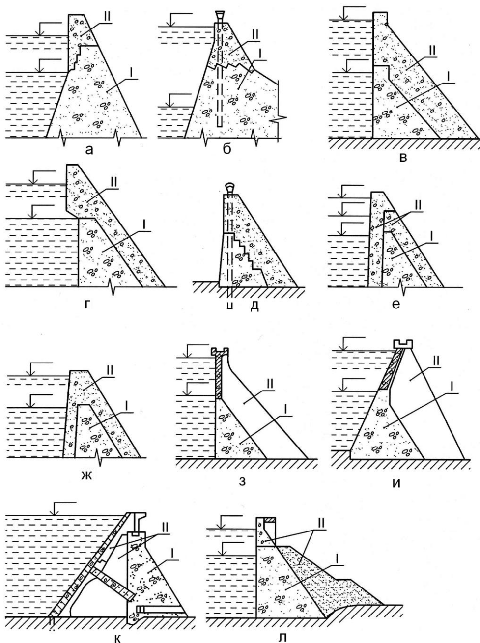
4.11. - расм. Реконструкцияда гравитацион тўғонларни ўстириш схемалари: I – эски тўғон; II – тўғонни ўстириш (қучайтирадиган) конструкциялари.
