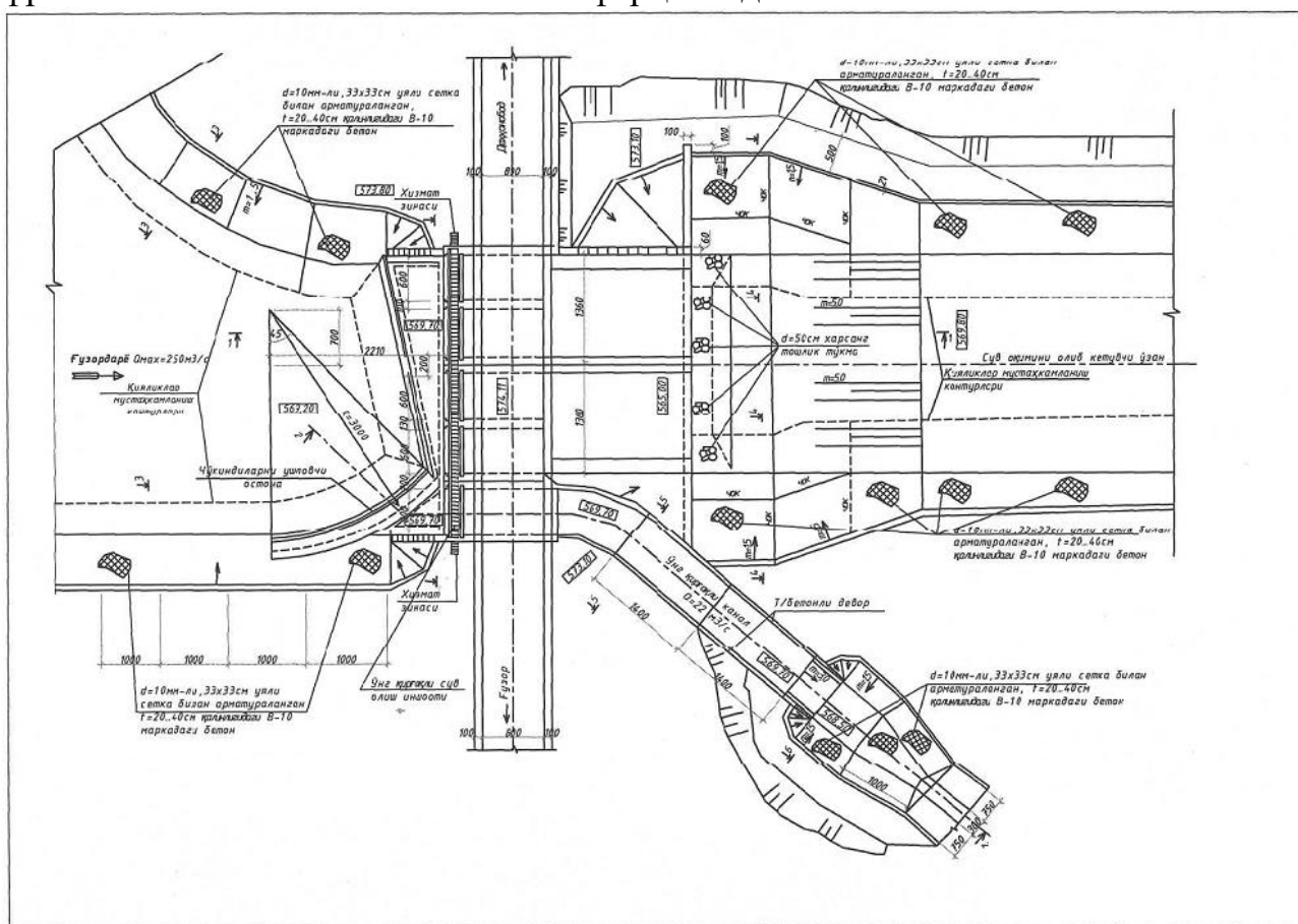
2.10. – расм. Фронтал дарёдан сув олиш гидроузели (Ғузор гидроузели) плани.
