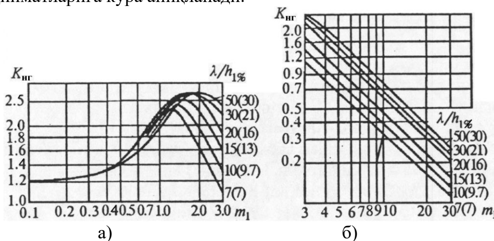
3 - расм. K_{nr} коэффициенти қийматларини аниқловчи графиклар: а) – m_1 \leq 3 бўлганда, б) – m_1 \geq 3 бўлганда.
