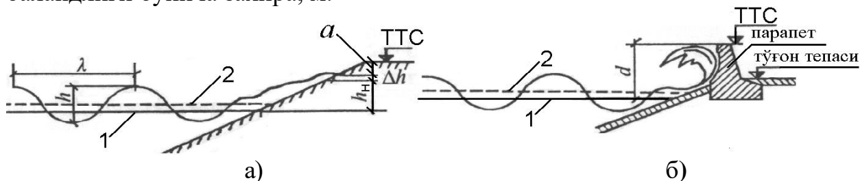
1 - расм. Тўғон тепаси белгисини аниқлаш схемаси: а) — парапетсиз; б) — парапетли; 1 — ҳисобий статик сатҳ; 2 — ўртача тўлқин чизиғи, h - тўлқиннинг баландлиги, \lambda - тўлқиннинг узунлиги.
