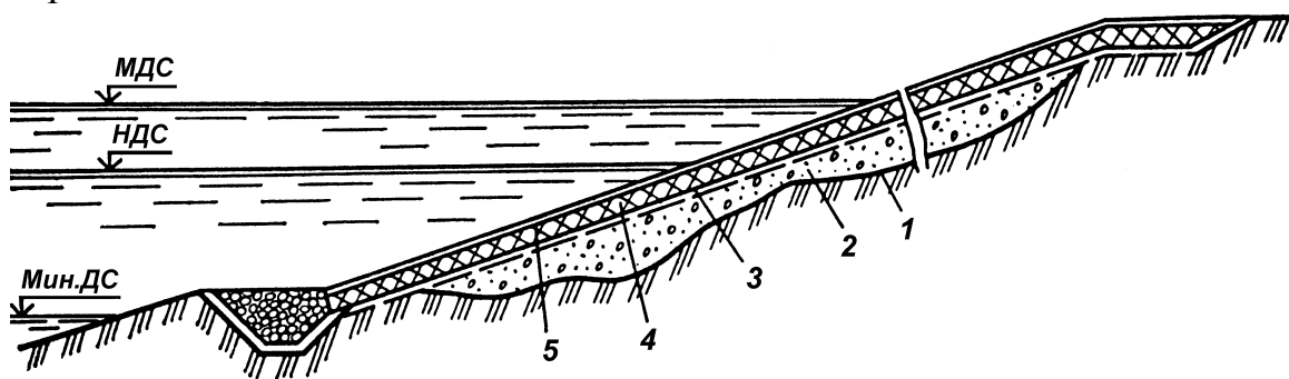
3.11. – расм. Асфальтбетон қопламаси билан грунтли тўғоннинг қиялигини қайта тиклаш: 1 - қияликнинг бузилган чегараси; 2 – қум-гравийлик грунт билан тўлдирилган қисми, 3 – захарли кимё моддалари билан едирилган зонаси, 4 – асфальтбетонлик қоплама; 5 – ишлов берилган юза.
