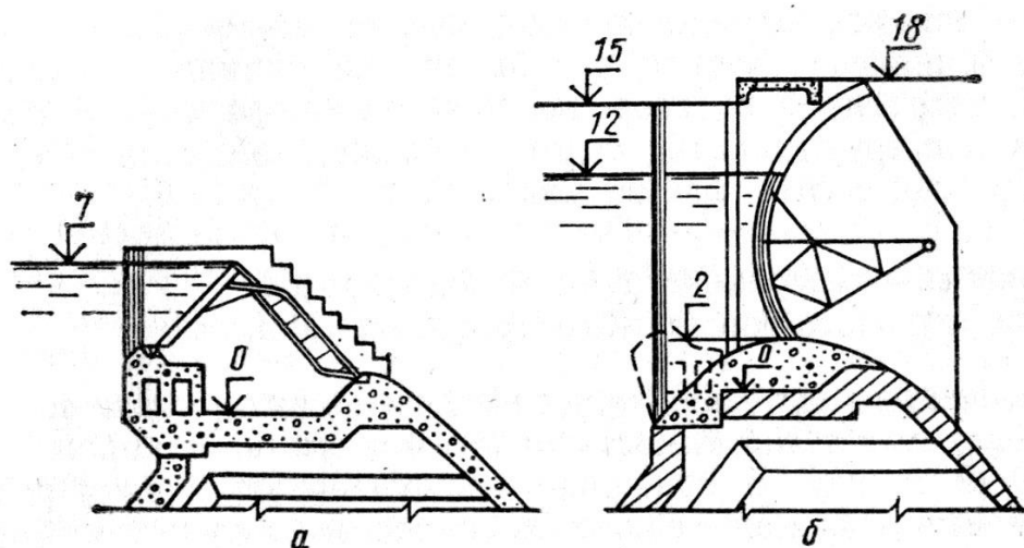
4.13. - расм. Поссум - Кингдом тўғонини реконструкция схемаси: а ва б - реконструкциягача ва ундан кейинги оқова ва затворлар
