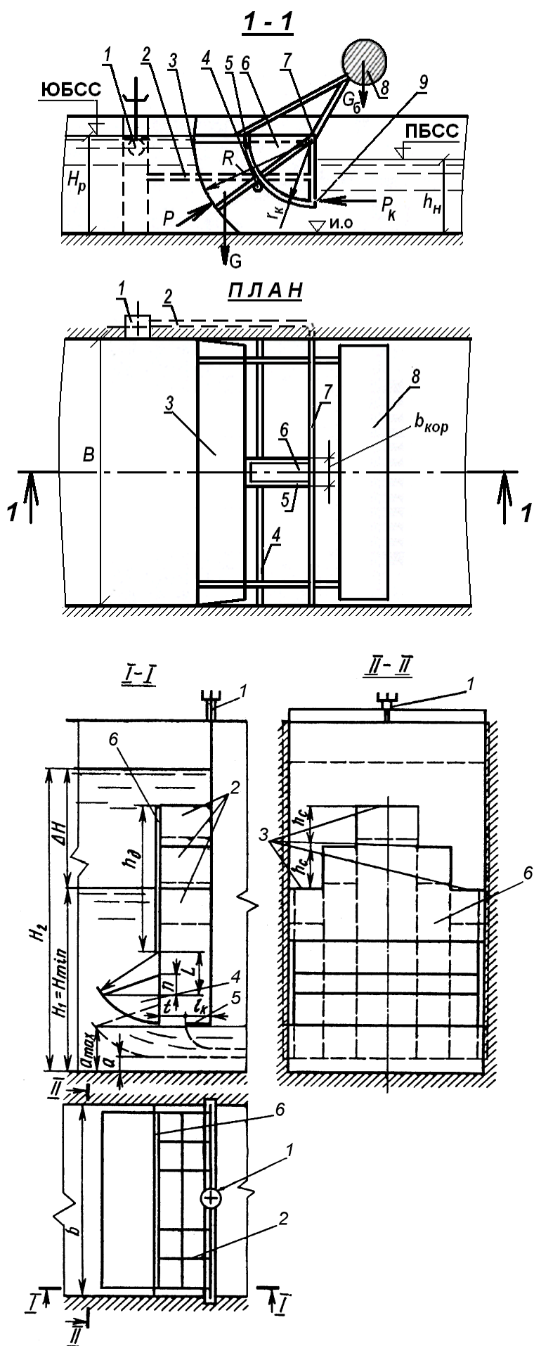
2.17. – расм. Я.В. Бочкарев таклиф этган корректорлик камераси ёрдамида тўғри ишловчи мувозанатланган сув сатҳини бошқарувчи сегментли затвор - автомат конструкцияси: 1 - сув сатҳини белгиловчи датчик; 2 - сув келтирувчи қувур; 3 - затвор - автоматнинг қобиқи; 4 - таянчлик тўсин; 5 - корректорлик камераси; 6 - корректор; 7 - шарнир; 8 - балансир; 9 - сув чиқарувчи тешик.
