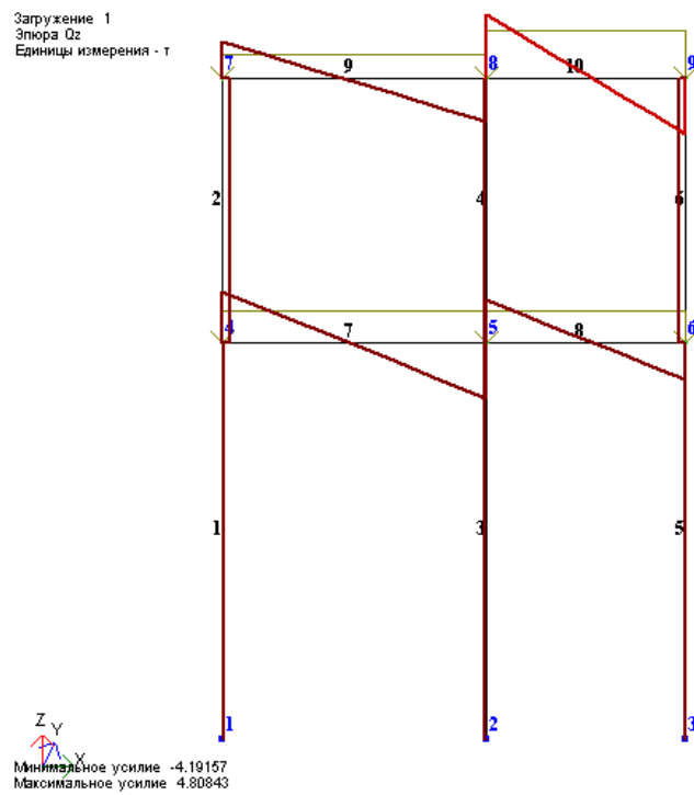
18-расм. Q_z кўндаланг кучлар эпюраси
