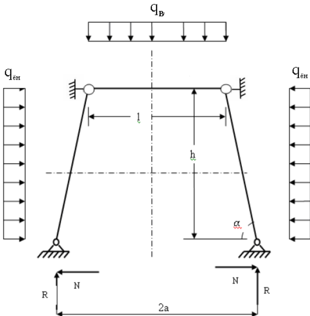
22-расм. Шарнирли раманинг ҳисоб схемаси
