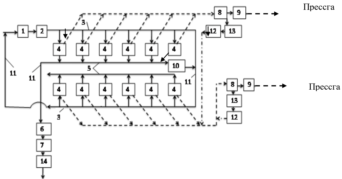
8-расм. 1ВПУ (2ВПУ) тўғри оқимли бир цилиндрли тола тозалагиччи 4ДП-130 (5ДП-130) жинлар қатори пневмотранспорт тизимининг схемаси
