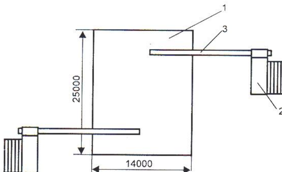
1- ғарам майдони; 2- ХПП-III қабул қилиш қурилмаси; 3-КЛП-650 транспортери
