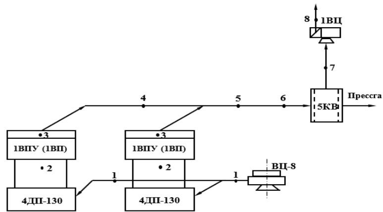
8-расм. 1ВПУ (2ВПУ) тўғри оқимли бир цилиндрли тола тозалагиччи 4ДП-130 (5ДП-130) жинлар қатори пневмотранспорт тизимининг схемаси
