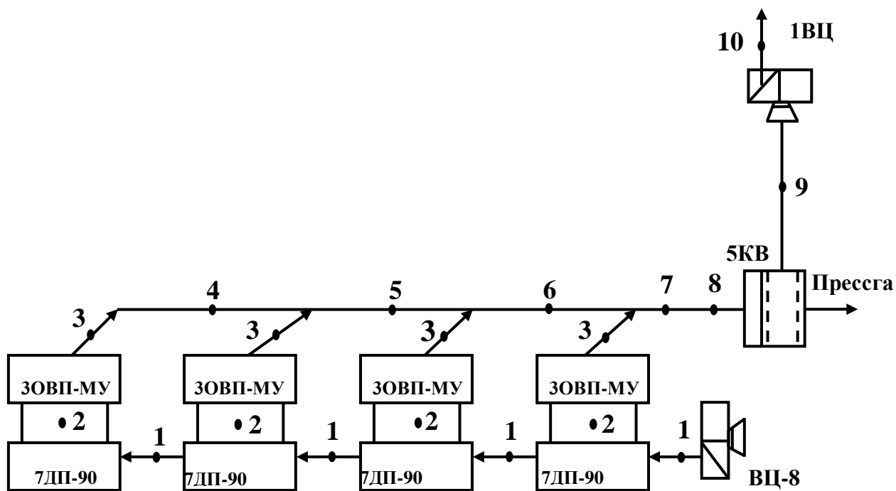
7-расм. 3ОВП-МУ тўғри оқимли бир цилиндрли тола тозалагичли 7ДП-90 жинлар қатори пневмотранспорт тизимининг схемаси
