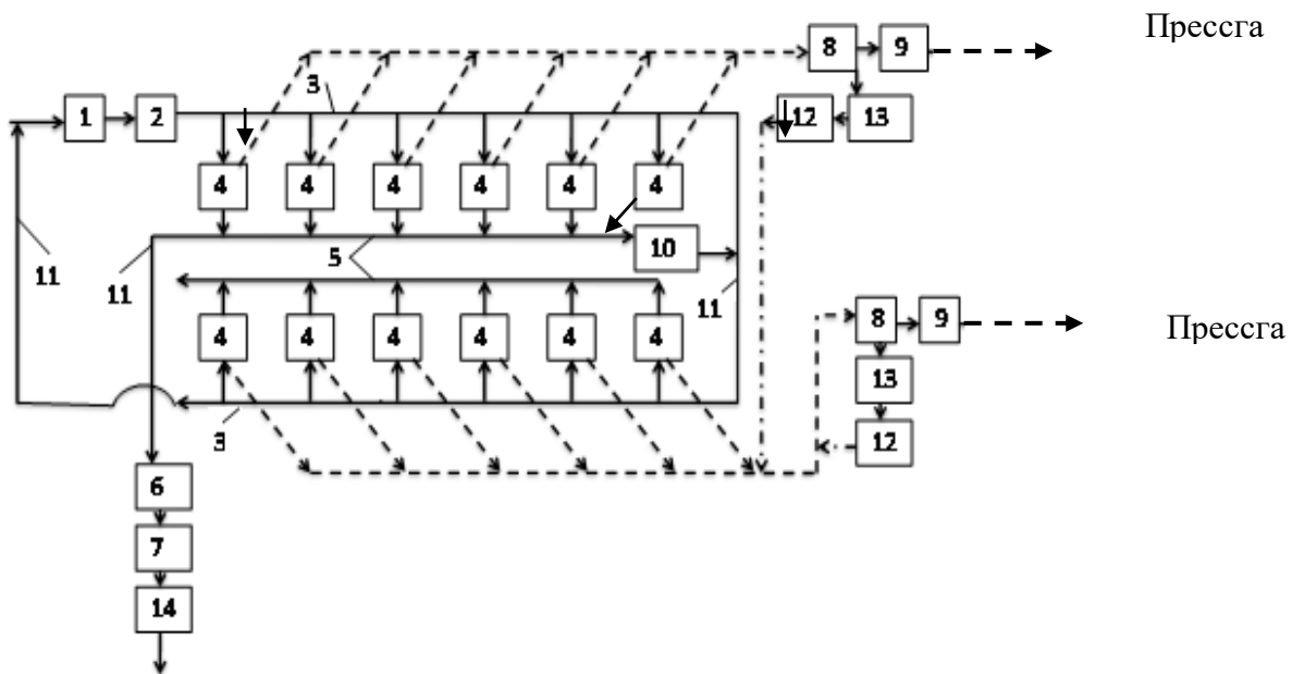
8-расм. 1ВПУ (2ВПУ) тўғри оқимли бир цилиндрли тола тозалагичли 4ДП-130 (5ДП-130) жинлар қатори пневмотранспорт тизимининг схемаси
