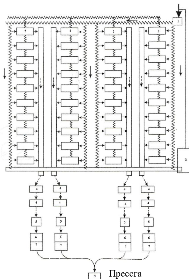
10-расм. Момикли чиқиндидан калта штапелли момик ажратиш олиш жараёни схемаси
