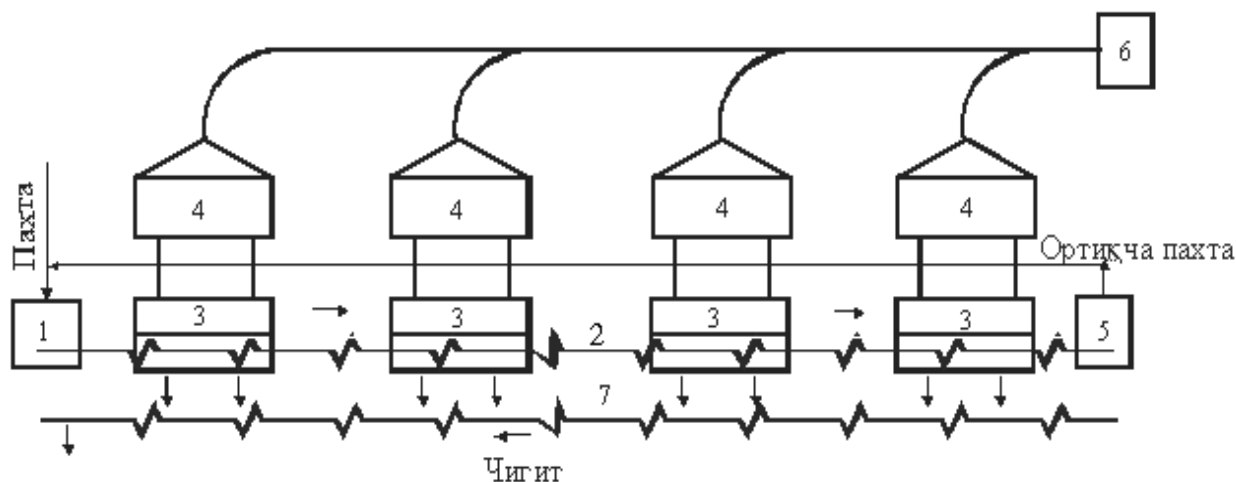
4-расм. ДПЗ-180 русумли 2 та жинли пахта тозалаш корхонаси бош корпусининг жинлаш бўлимида технологик ускуналарнинг жойлашиш таркиби ва кетма-кетлиги
