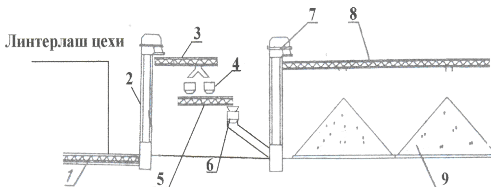
1, 3, 5, 8- винтли конвейерлар; 2, 7- элеваторлар; 4- тарози; 6- 3С русумли қурилма; 9- чигит
