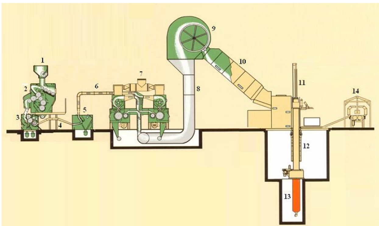
4.1-расм Пахта толасини жинлаш, тозалаш ва тойлашни технологик ускуналарнинг жойлашув кетма-кетлиги
