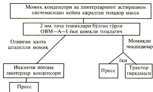
10-расм. Момикли чиқиндидан калта штапелли момик ажратиш олиш жараёни схемаси
