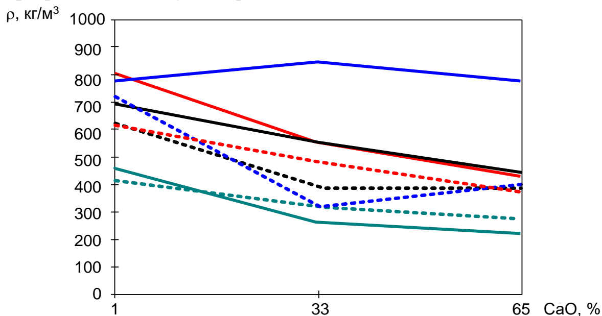
1.1.-расм. Газобетонларнинг зичлиги: кварцликум (тўққўк); ИЭС кули (қора); туф (қизил); микрокремнезем (хаворанг) асосдаги. Пунктирли чизиқлар - фиброгазобетон учун
