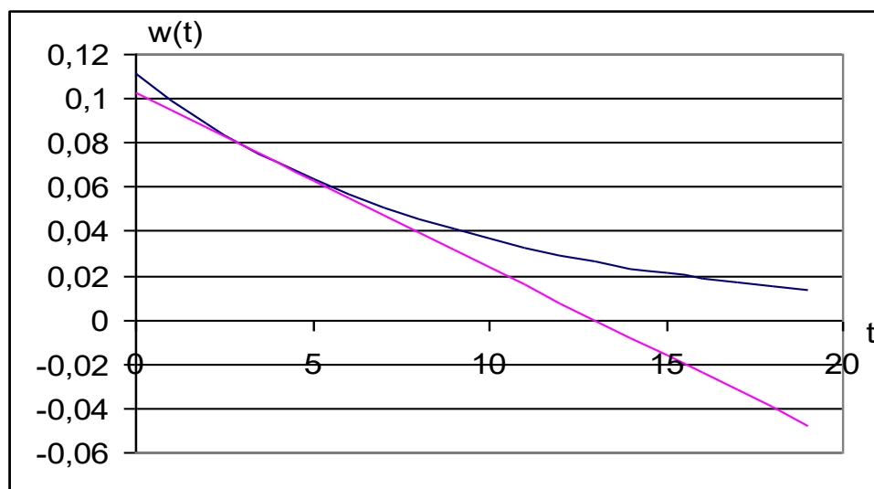
Рис. 7. Определение постоянное времени из весовой функции
