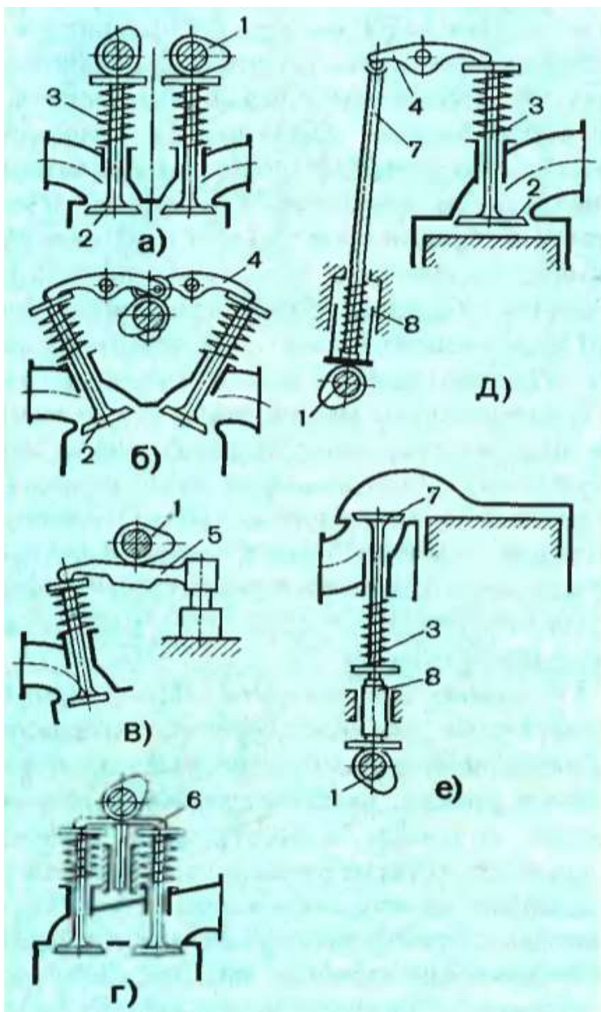
5-расм. Клапанларни ўрнатиш ва уларни ҳаракатга келтириш учун қўлланилган газ тақсимлаш механизми схемалари:
