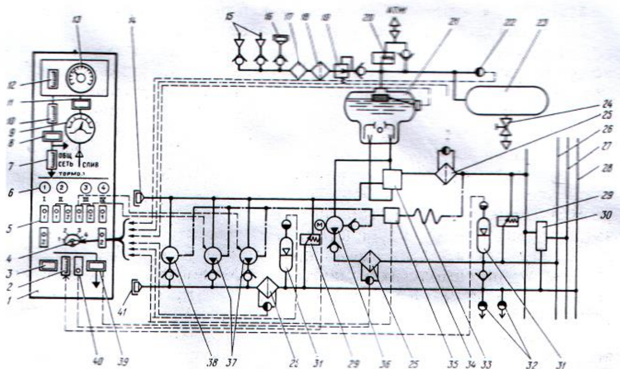
Рис 6. Схема сети источников давления и панель гидросистемы.
