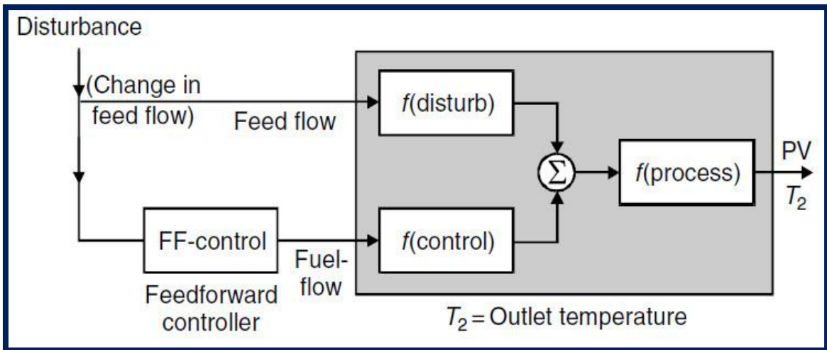
Рис. 2.4. Предупреждение блок- схема
