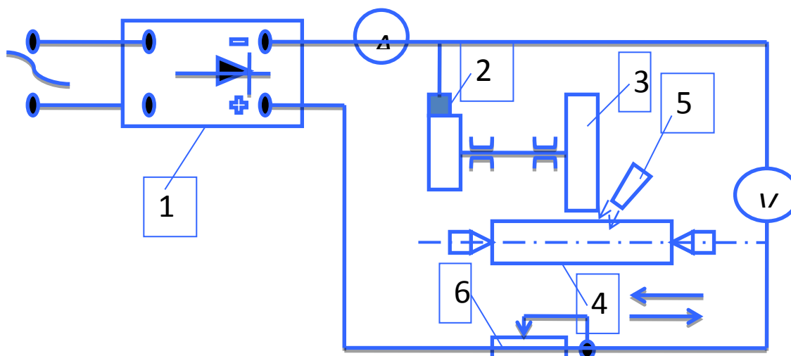
2- rasm. Elektroabraziv ishlashni prinsipl sxemasi. 1 - doimiy tok manbai; 2 - sirpanuvchi kontakt; 3 - tok utkazuvchi jilvir tosh; 4 - ishlanayotgan detal; 5 - elektrolit; 6 - reostat.
