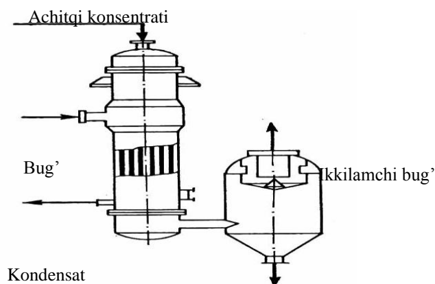
расм. Қатламли оқиб келувчи бујлантириш ускунаси.
