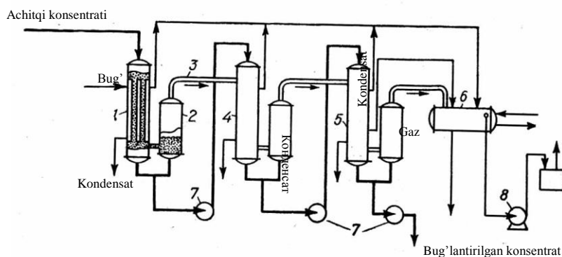
расм. Уч корпусли бујлантириш ускунаси:
