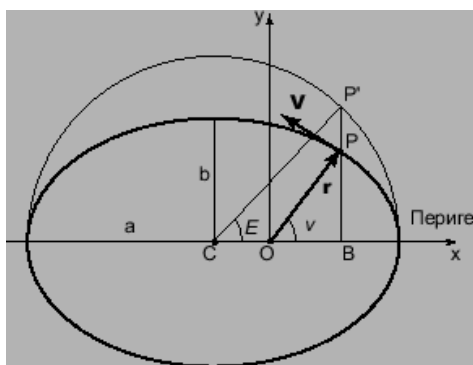
7-расм. Кеплер орбитасининг аномалиясини аниқлаш
