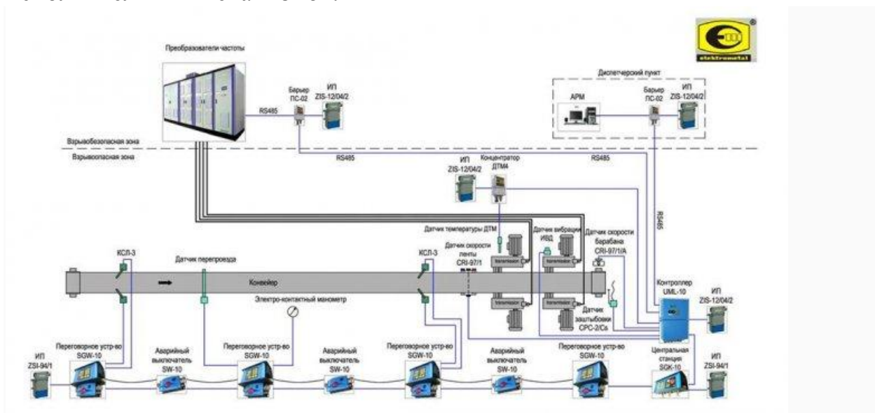
Рис. 2.2. - Структурная схема системы
