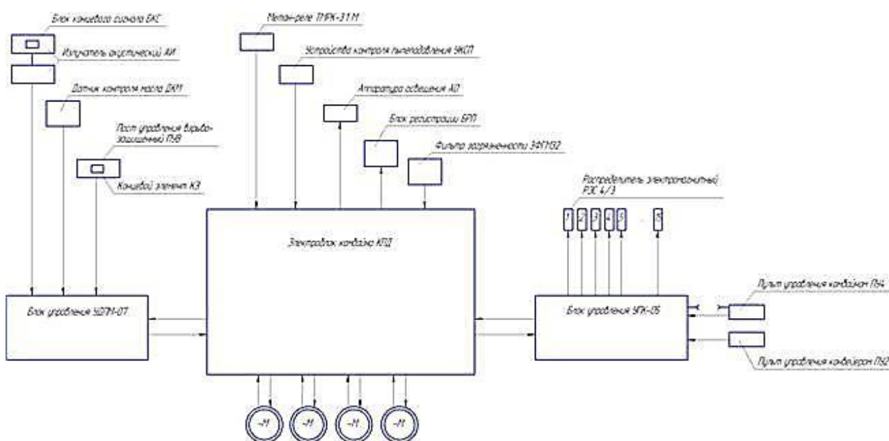
Рис. 1.2 - Структурная схема комбайна КПД
