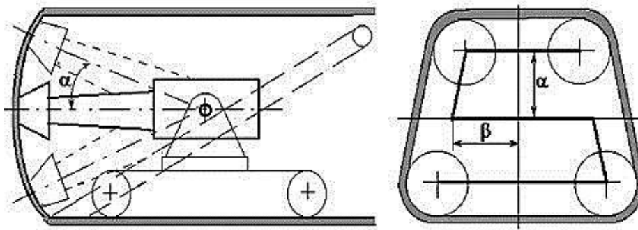
Рис.1.4. Схема проходки выработки трапециевидного сечения комбайном со стреловым исполнительным органом.
