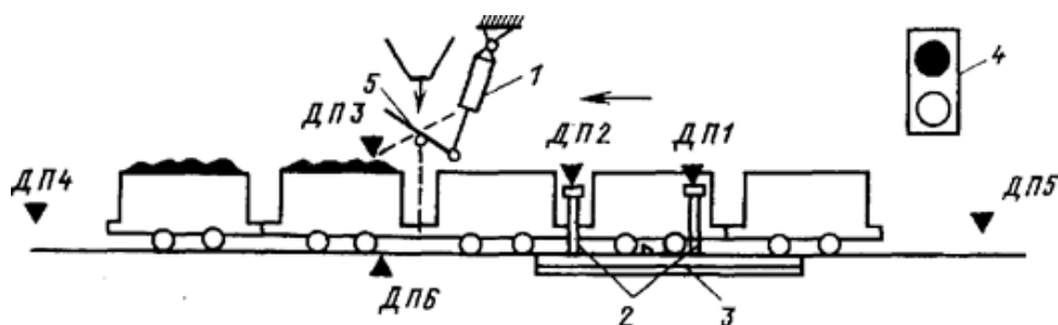
Рис.2.6 - Технологическая схема автоматизированного погрузочного пункта
