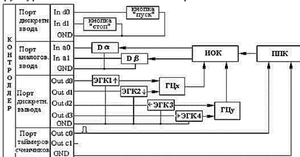
Рис.1. 5. Структура системы автоматического управления траекторией
