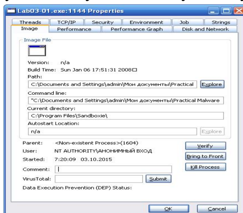
4.6-расм. Process Explorer дастурий воситаси хусусиятлар ойнаси
