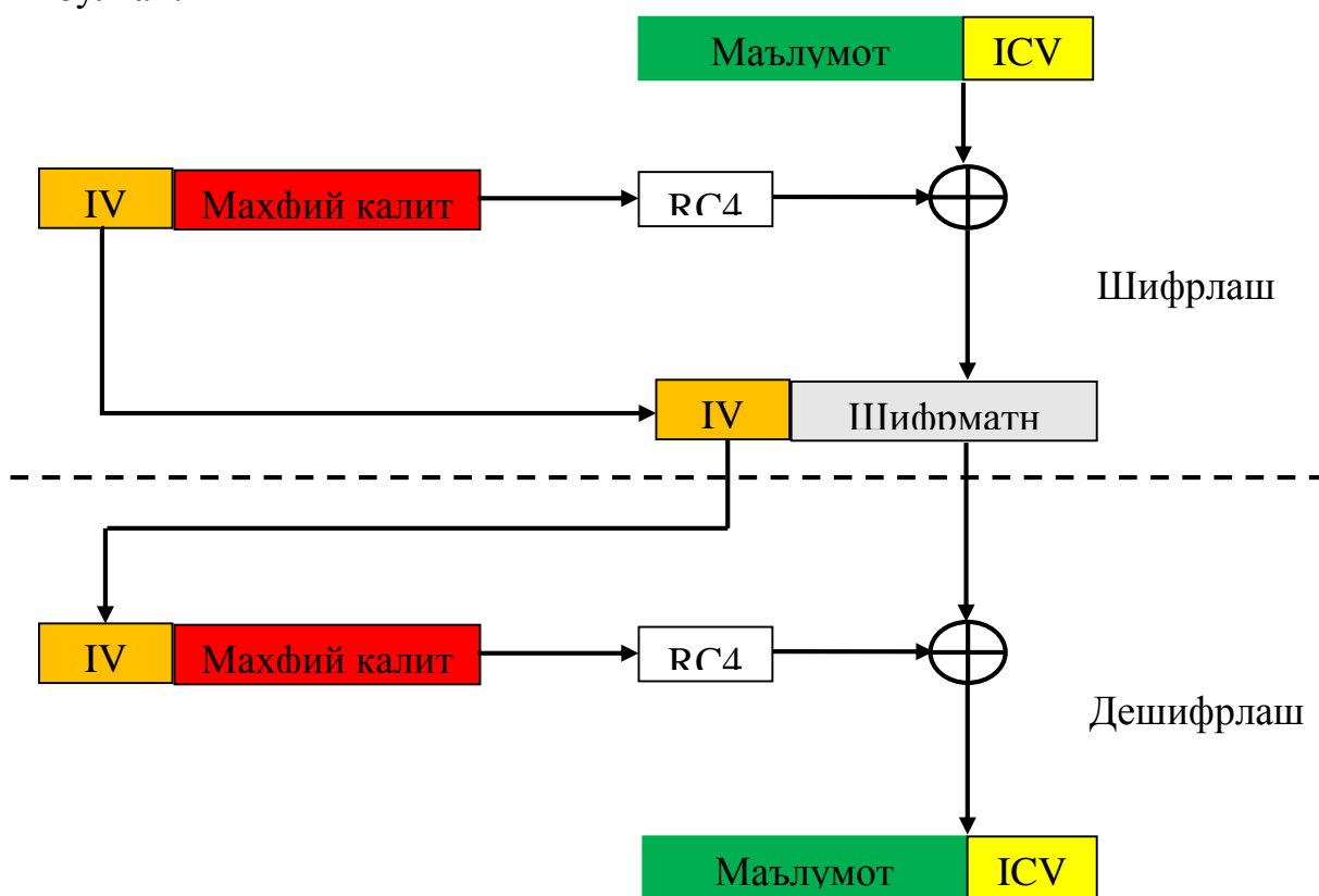
3.56-расм. WEP протоколида шифрлаш
