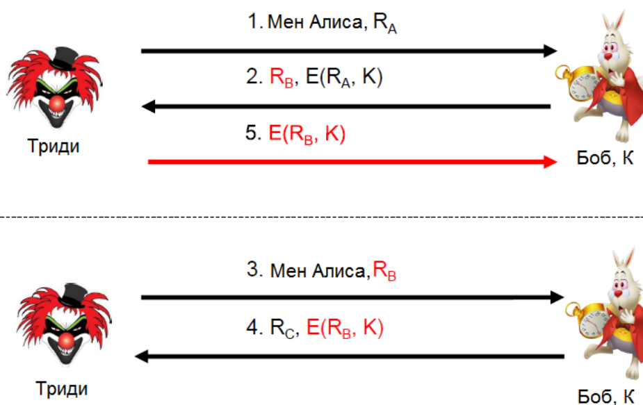
3.10 – расм. Пареллел сеанс асосида таҳдид
