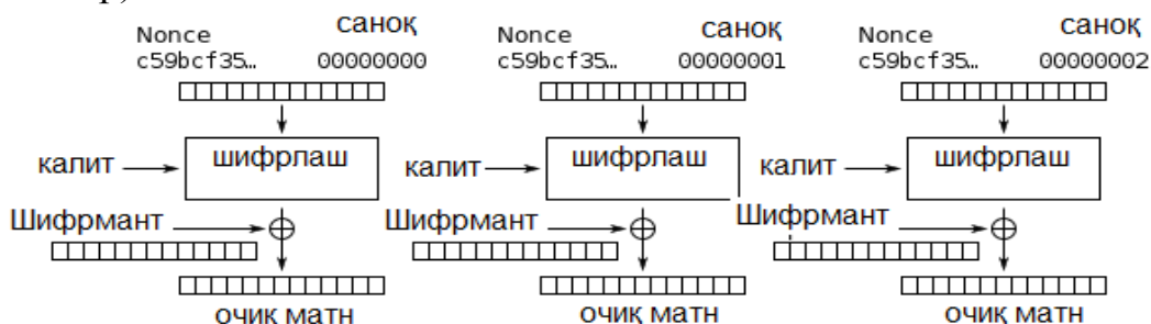
1.17-расм. CTR моделда дешифрлаш
