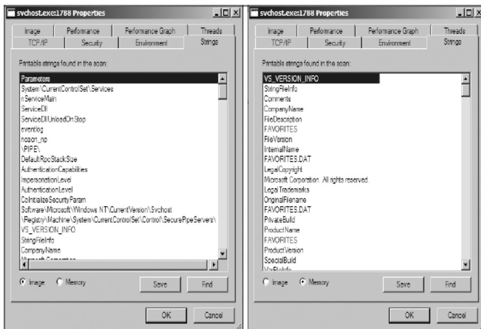
4.7-расм. Қаторларни солиштириш
