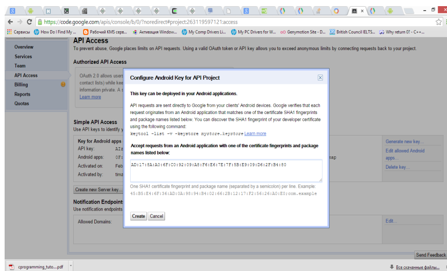
4.10-расм. Лойиҳа учун Google API калитини олиш
