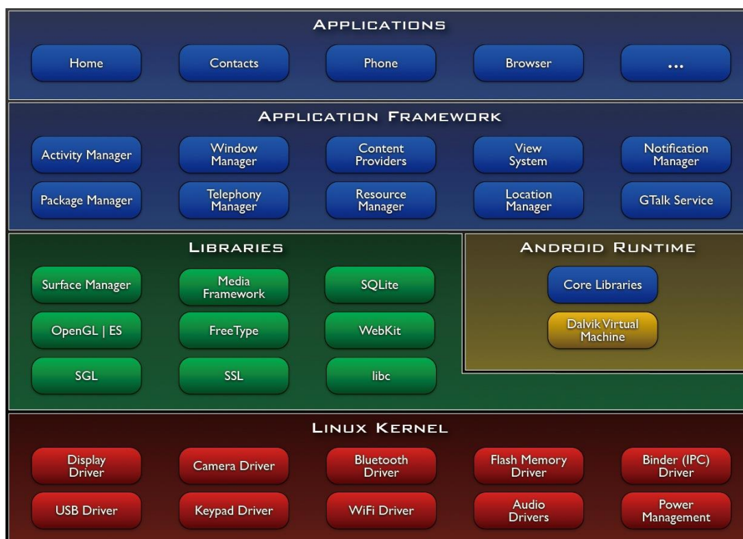
1.2-расм. Андроид ОТ архитектураси
