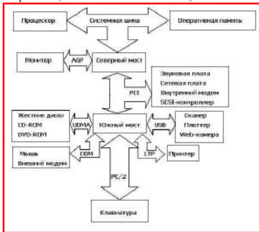
Рис. 1 Логическая схема системной платы
