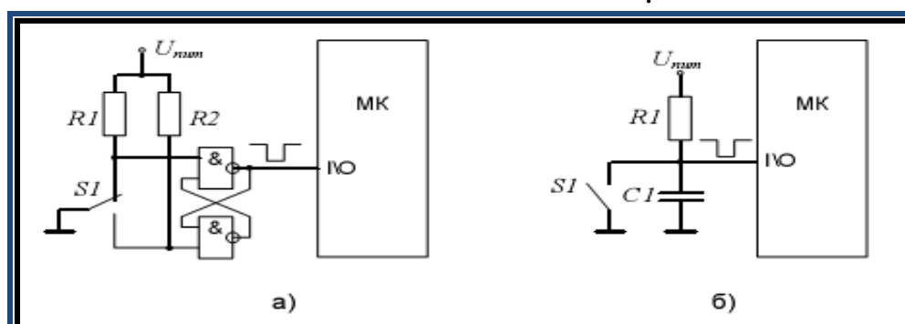
Рис. 7 Способы аппаратного подавления дребезга контактов
