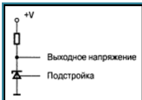
Рис. 2 ИС LM335
