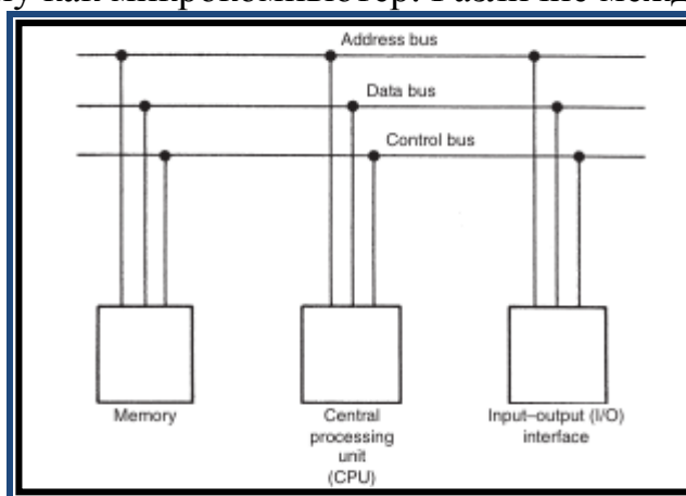
Рис. 1 Элементы микрокомпьютера
