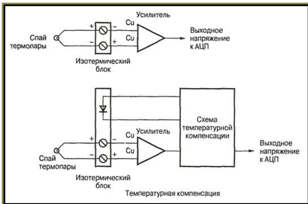
Рис. 1 Термопара
