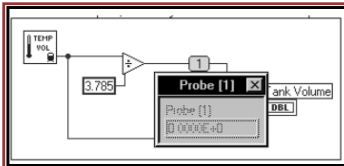
Рис.40 Блок-схема
