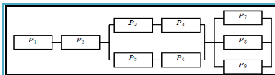
Рис.4 Структурная схема надежности технической системы
