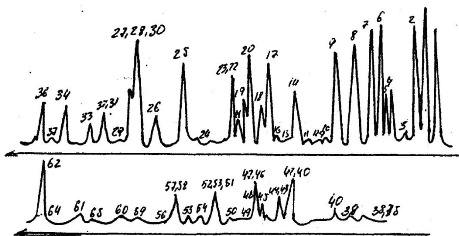
5-расм. Узушлиги 150 м бўлган октадесен-1 фазали, 30 0 С да ушланган 125 0 С гача ҳароратда қайнаб кетувчи бензин фракциясининг хроматограммаси.
