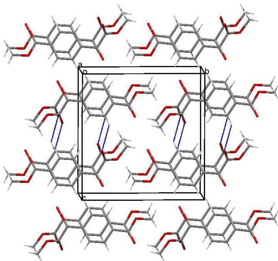
Рис.2. Кристаллическая структура IXб.
