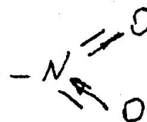
Асимметрик тебраниш
