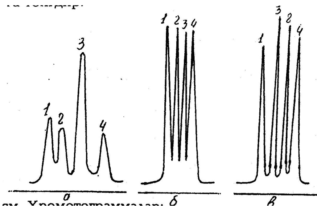
6-расм. Хроматограммалар:
