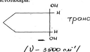
Хар хил турдаги гидроксил гуруҳларнинг ИК соҳадаги ютилиш частоталари:
