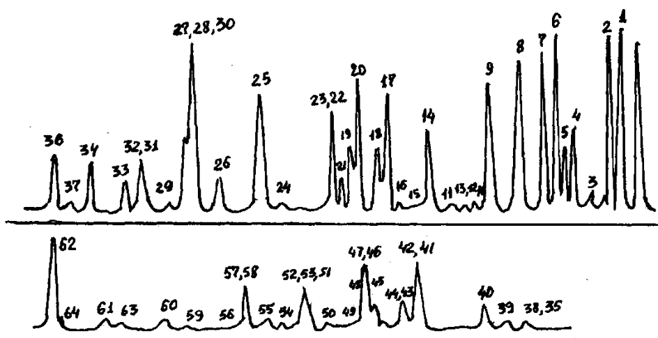
8-расм. Узунлиги 150 м бўлган октадецен–1 фазали, 30°С да ушланган 125°С гача ҳароратда қайнаб кетувчи бензин фракциясининг хроматографияси: 1–изопентан; 2–н–пентан; 3–2,2–диметилбутан; 4–циклопентан; 5–2,3–диметилбутан; 6–2–метилпентан; 7–3–метилпентан; 8–н–гексан; 9–метилциклопентан; 10–2,2–диметилпентан; 11–бензол; 12–2,4–диметилпентан; 13–2,2,3–триметилбутан; 14–циклогексан; 15–3,3–диметилпентан; 16–1,1–диметилциклопентан; 17–2–метилгексан; 18–2,3–диметилпентан; 19–цис–1,3–диметилциклопентан; 20–транс–1,2–диметилциклопентан; 23–3–этилпентан; 24–2,2,4–триметилпентан; 25–н–гептан; 26–цис–1,2–диметилциклопентан; 27–метилциклогексан; 28–этилциклогексан; 29–2,2,3,3–тетраметилбутан; 30–2,2–диметилгексан; 31–
