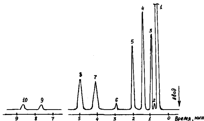
13-расм. Таркибида водород сульфид, карбонат ангидрид, метаноли бўлган табиий газни компонентларга ажралиши: 1-метан; 2-карбонат ангидрид; 3-этан; 4-водород сульфид; 5-пропан; 6-метанол; 7-и-бутан; 8-н-бутан; 9-и-пентан; 10-н-пентан.
