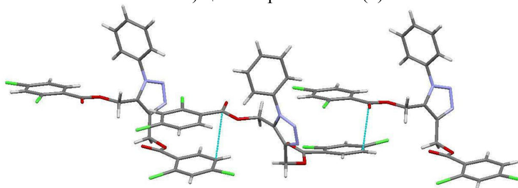
рис.2. Ассоциаты образующих \pi - \pi стэкинг взаимодействиями в кристаллической структуре дихлатазола
