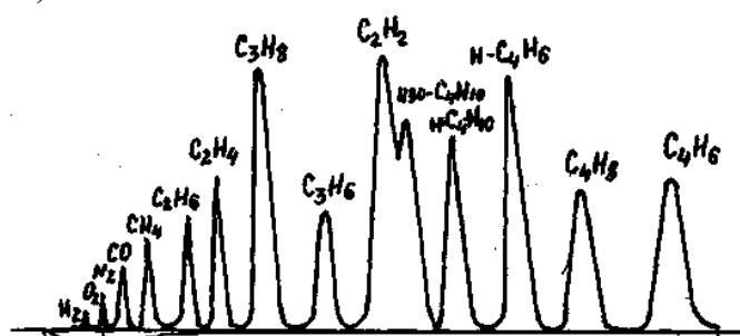
12-расм. Куйи углеводородларни алюмогельда ажралиши (колонканинг узунлиги–6,6м).
