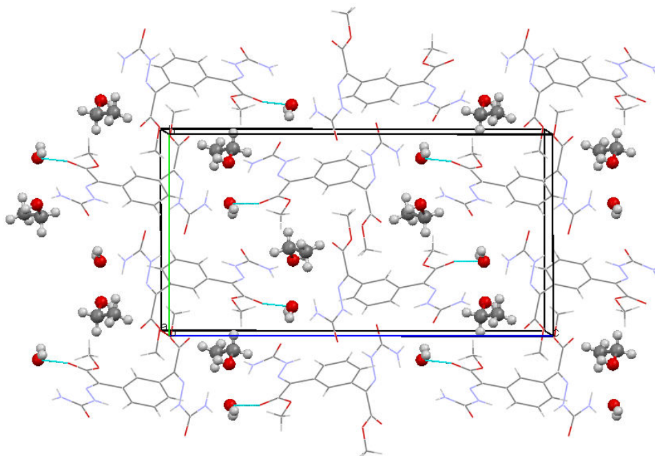
Рис.4. Кристаллическая структура моногидрата сольвата дисемикарбазона диметилового эфира 1,3-бензолдикетодикарбоновой кислоты с этанолом
