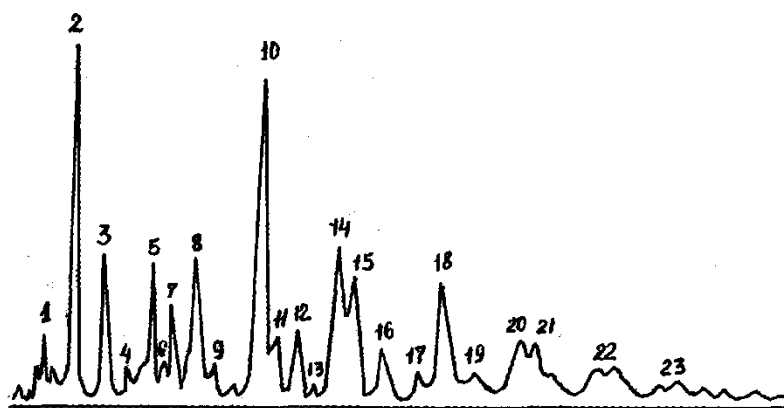
10 расм. Тошкўмир мойи хроматограммаси: 1–инден; 2–нафталин; 3–метилнафталин; 4–дифенил; 5–диметилнафталин; 6–аценафтен; 7–дифениленоксид; 8–флуорен; 9–метилфлуорен; 13–2-фенилнафталин; 14–флуорантетрацен; 20–бензофлуорантен; 21–бензофирен ÷ перилен; 22–пицен; 23–коронен.
